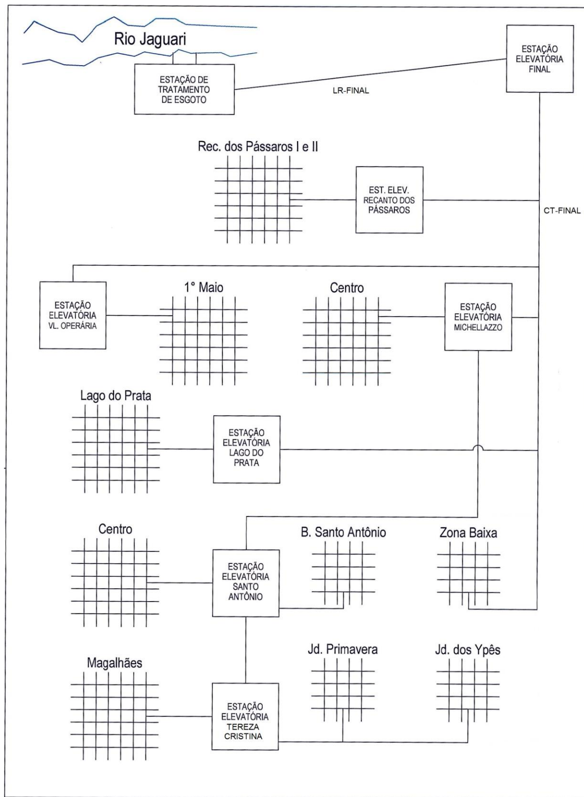
Figura 4.2 - Croqui do sistema de Esgotamento Principal
