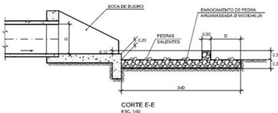
Ilustração 8.1 - Dissipador
