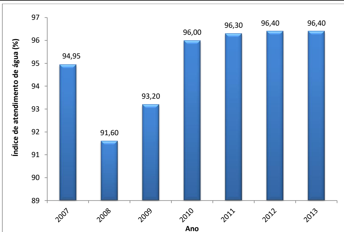
Gráfico 2.3 – Índice de Atendimento de Água
