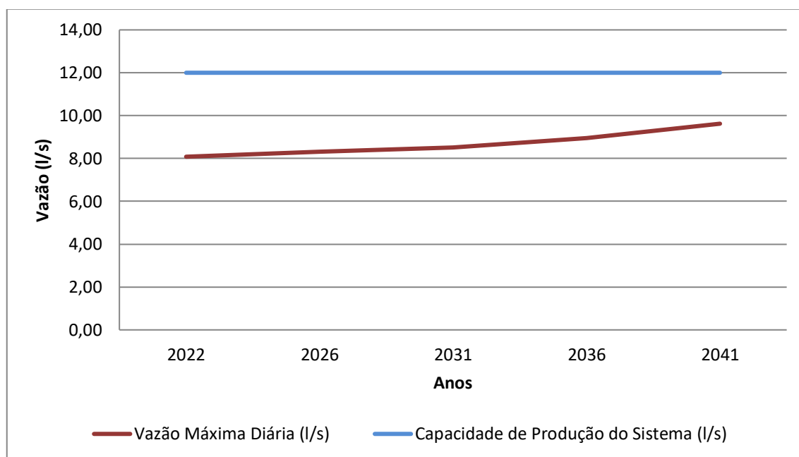
Gráfico 8.3 – Demandas Máximas Diárias (l/s) X Capacidade de Produção do Sistema (l/s)
