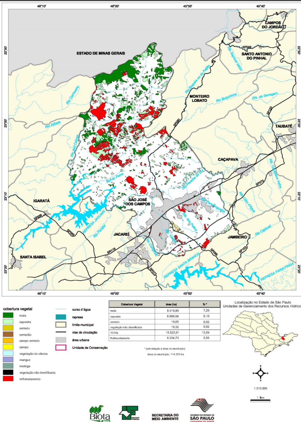
Figura 3.2 – Cobertura Vegetal no Município de São José dos Campos
