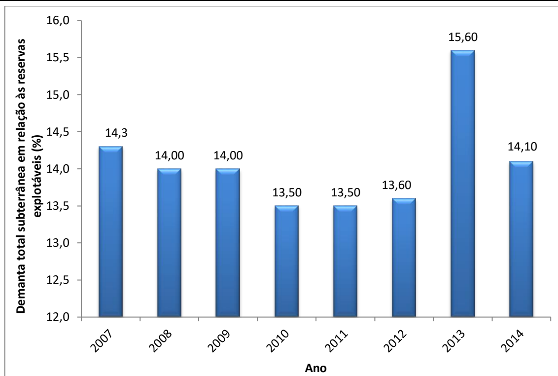
Gráfico 2.2 - Demanda Subterrânea em Relação às Reservas Explotáveis
