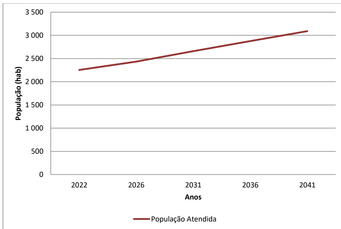
Gráfico 7.3 – População Atendida (hab.) x Anos de Planejamento – Distrito São Francisco Xavier
