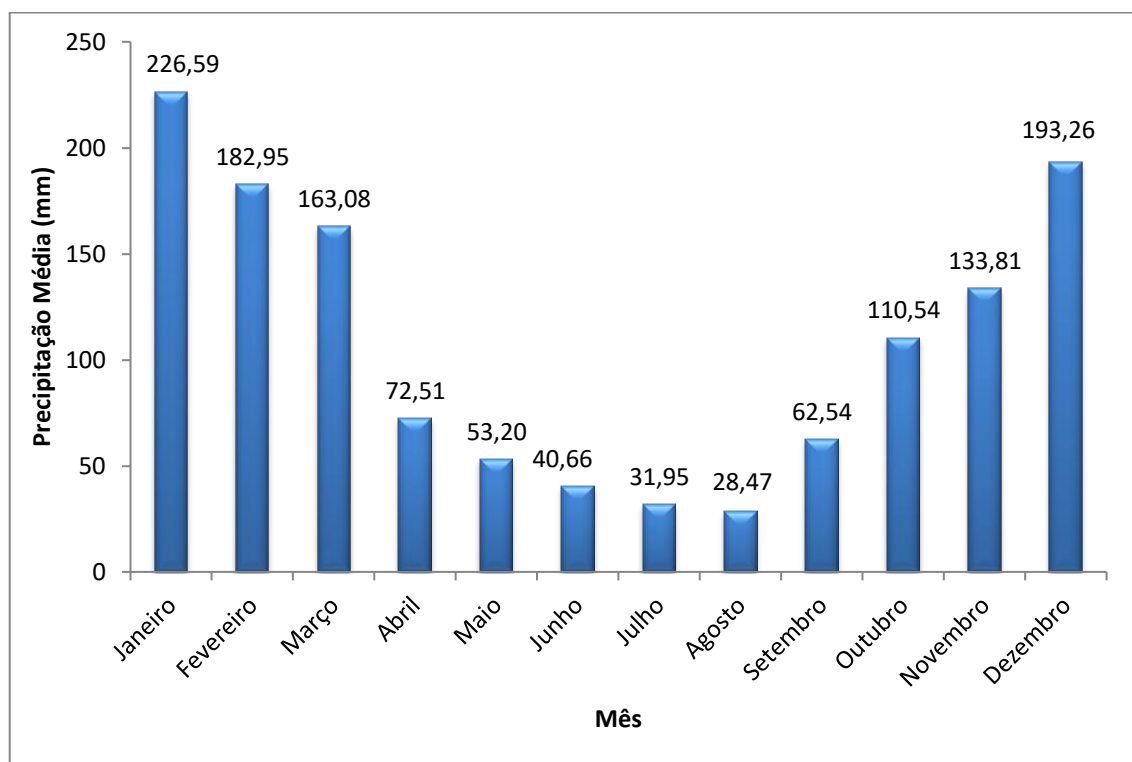
Gráfico 3.1 – Precipitação Média Mensal no Período de 1960 a 2021, Estação E2-099
