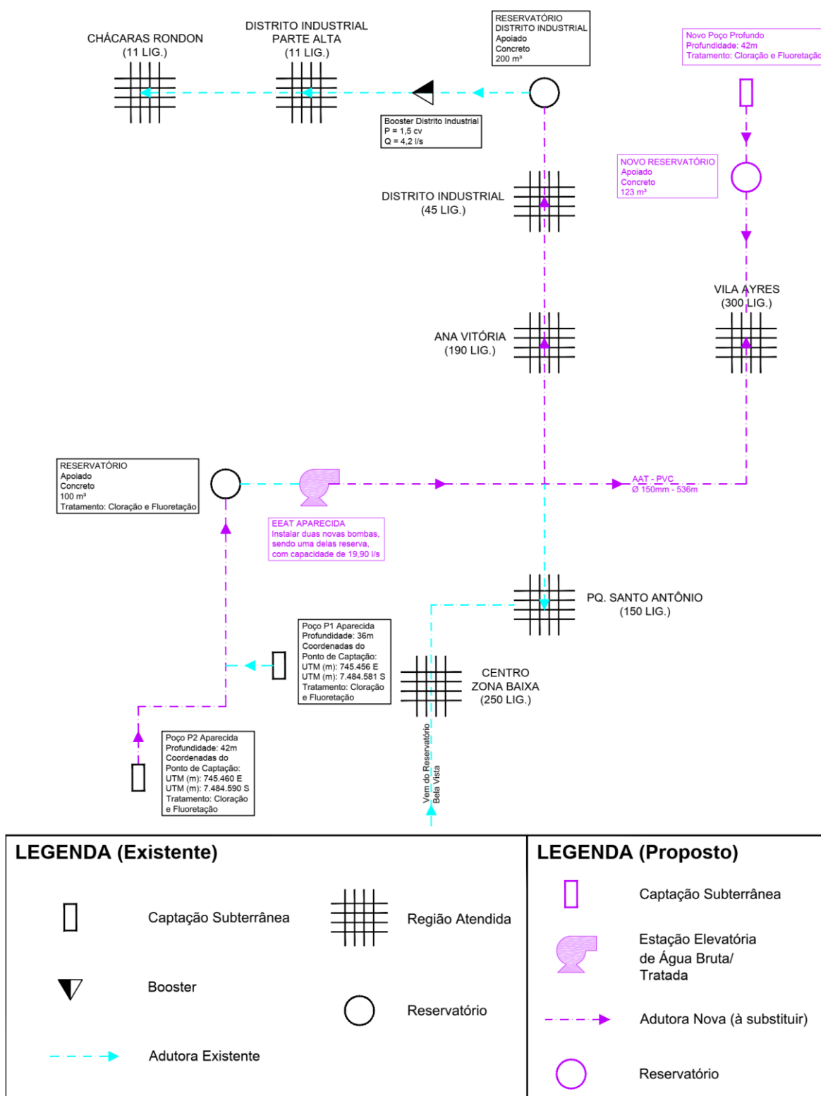
Figura 10.2 – Croqui do Sistema de Abastecimento de Água Proposto para o Sistema Distrito Aparecida de São Manuel
