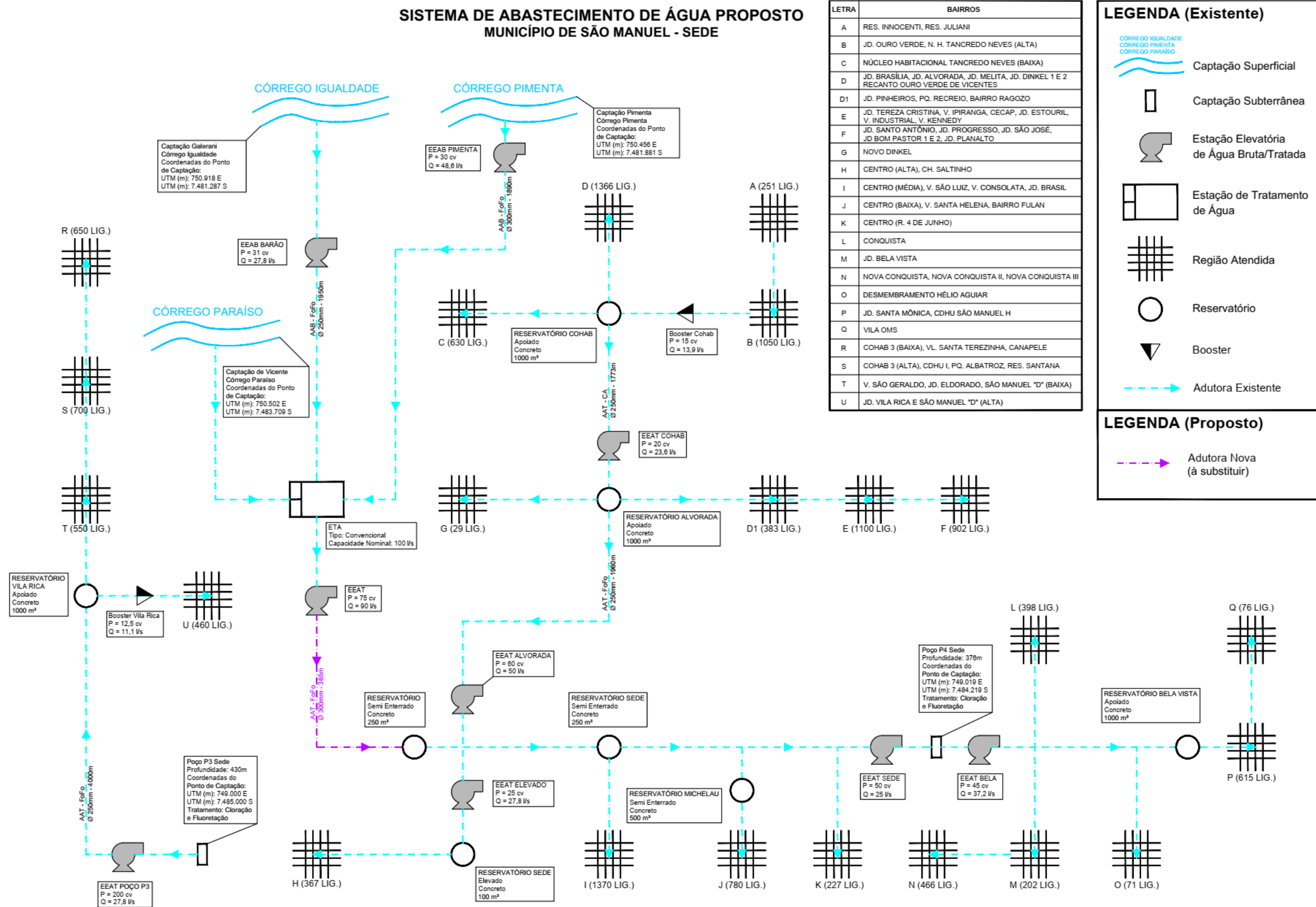
Figura 10.1 – Croqui do Sistema de Abastecimento de Água Proposto para o Sistema Sede Urbana
