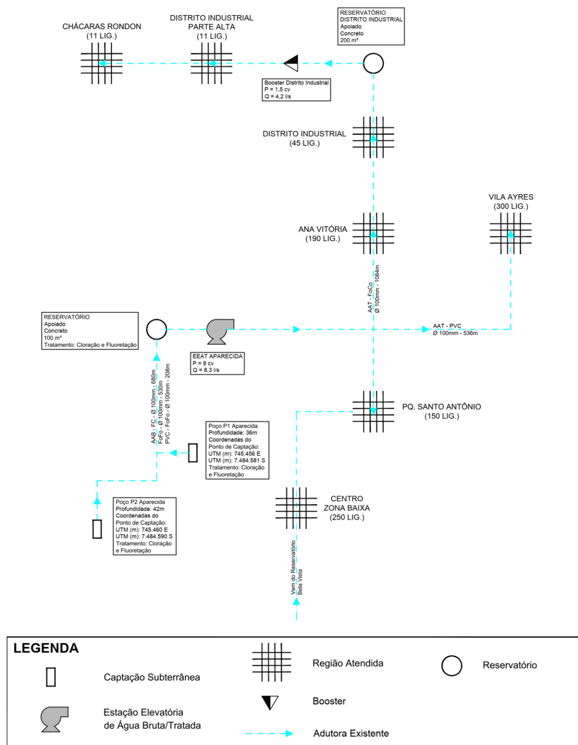
Figura 4.2 – Croqui do Sistema de Abastecimento de Água Existente – Distrito Aparecida de São Manuel.
