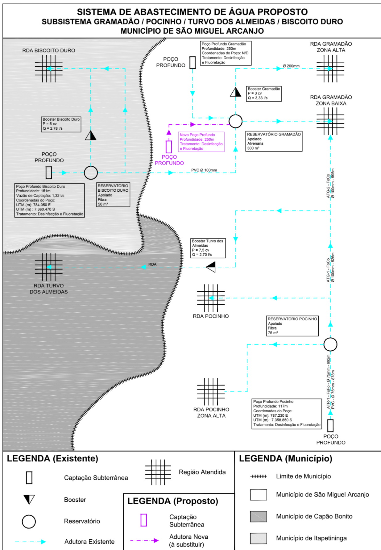
Figura 10.3 – Croqui do Sistema de Abastecimento de Água Proposto para os Bairros Gramadão/Pocinho/Turvo dos Almeidas/Biscoito Duro
