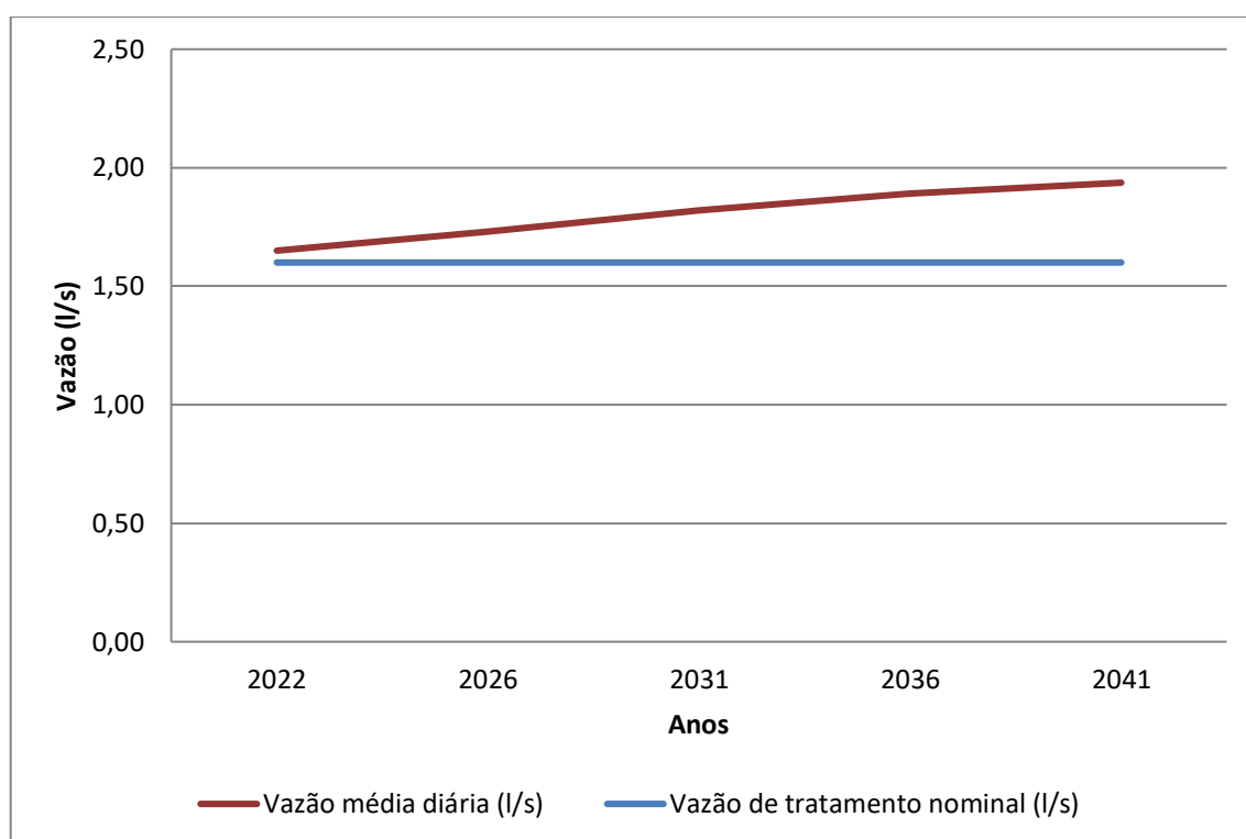
Gráfico 8.14 – Vazão Média Diária (l/s) x Capacidade nominal da ETE (l/s)
