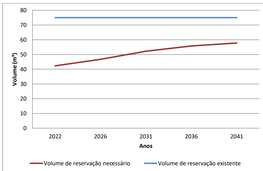
Gráfico 8.8 - Volume de Reservação Necessário (m³) x Volume de Reservação Atual (m³)
