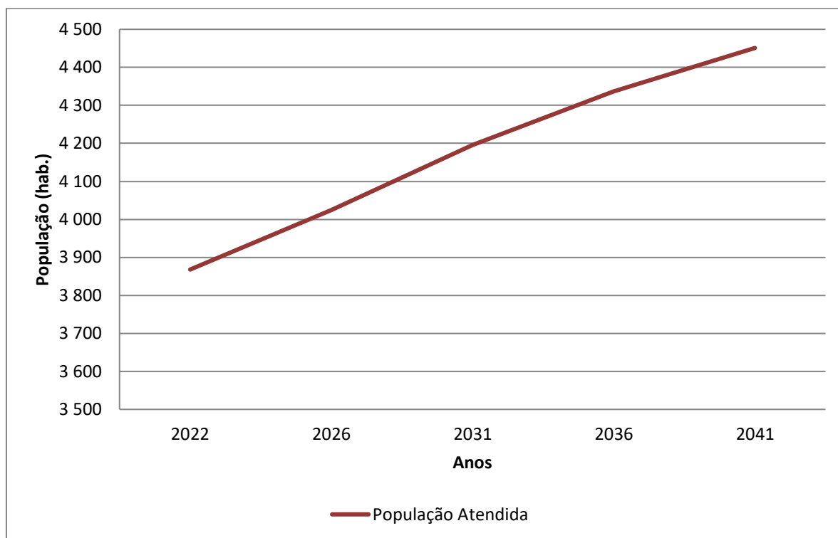
Gráfico 7.4 – População Atendida (hab.) x Anos de Planejamento – Bairros Gramadão/Pocinho/Turvo dos Almeidas/Biscoito Duro
