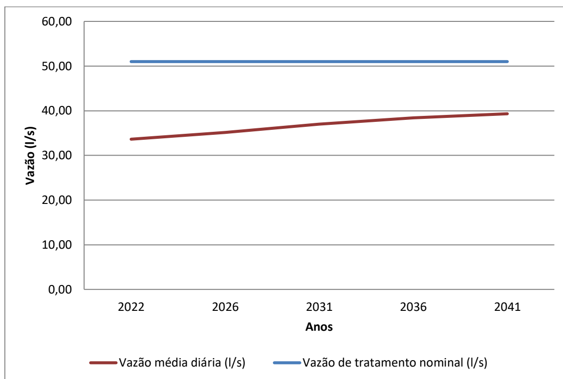
Gráfico 8.11 – Vazão Média Diária (l/s) x Capacidade nominal da ETE (l/s)
