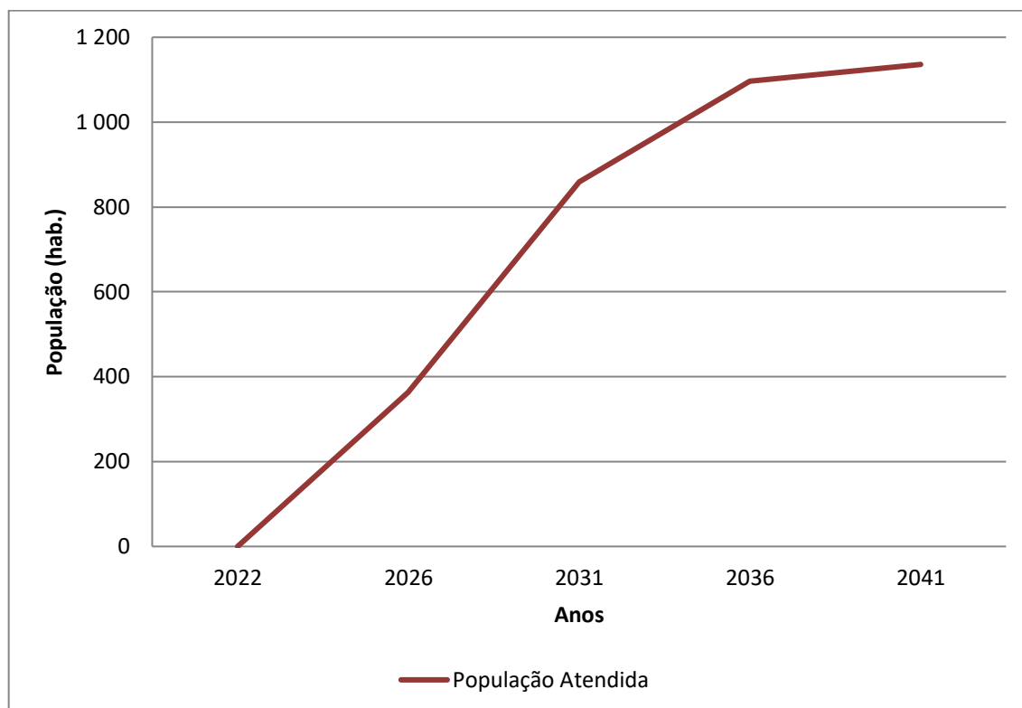
Gráfico 7.10 - População Atendida (hab.) x Anos de Planejamento – Bairros Abaitinga/Gaviões/Guararema
