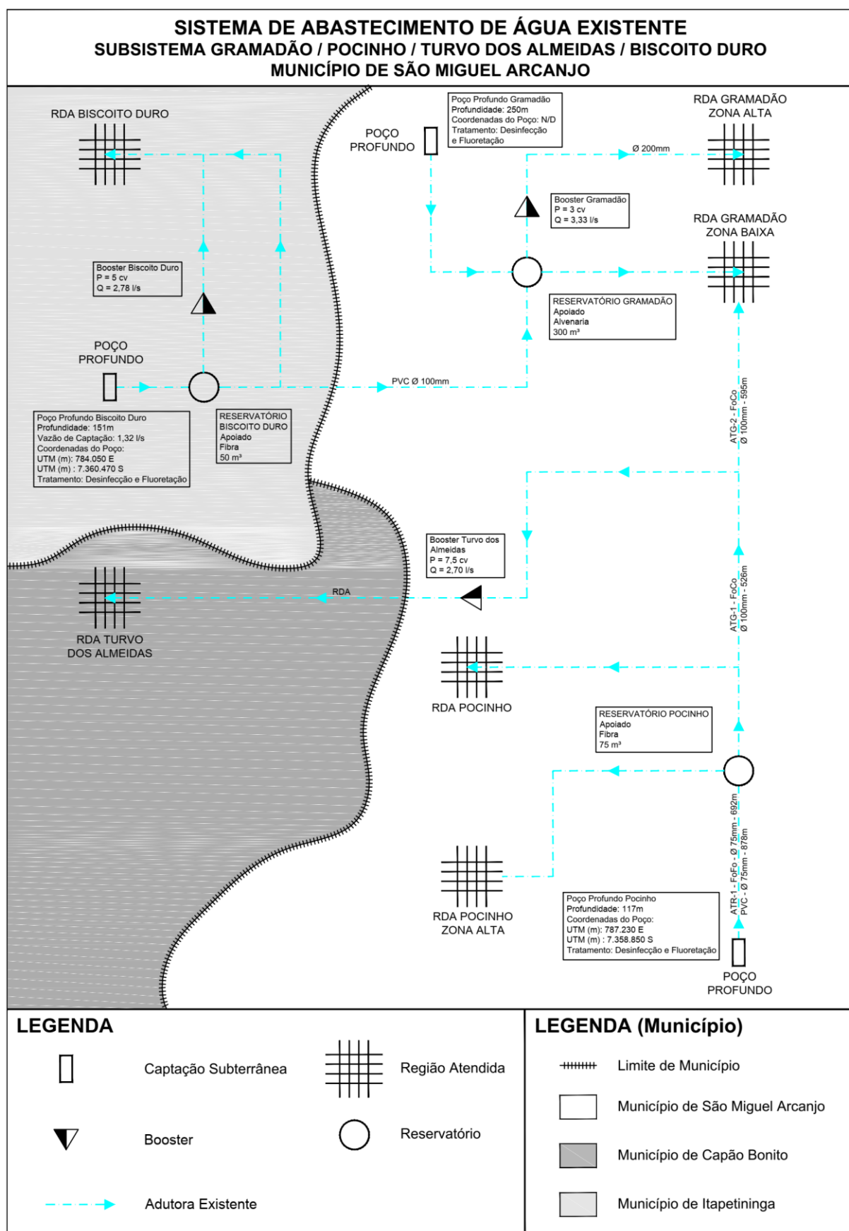
Figura 4.3 – Croqui do Sistema de Abastecimento de Água Existente – Bairros Gramadão/Pocinho/Turvo dos Almeida/Biscoito Duro.
