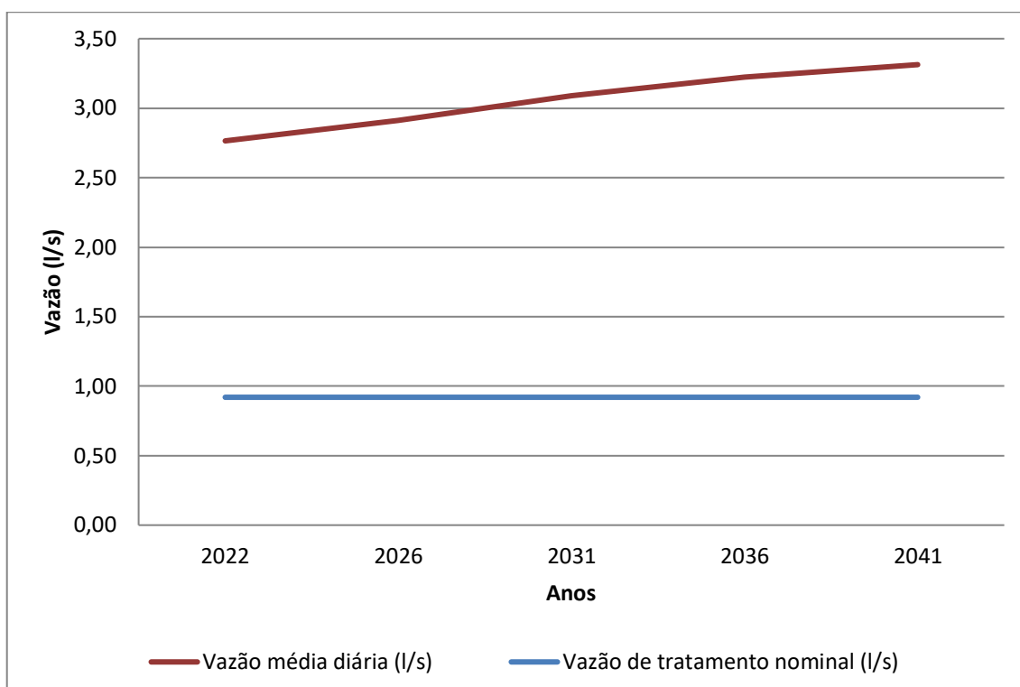
Gráfico 8.13 – Vazão Média Diária (l/s) x Capacidade nominal da ETE (l/s)
