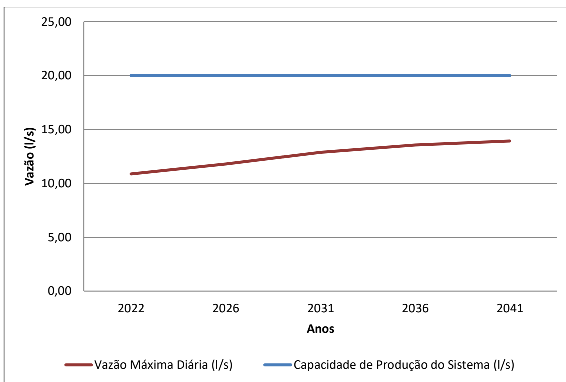
Gráfico 8.5 – Vazão máxima diária (l/s) x Capacidade de Produção do Sistema (l/s)
