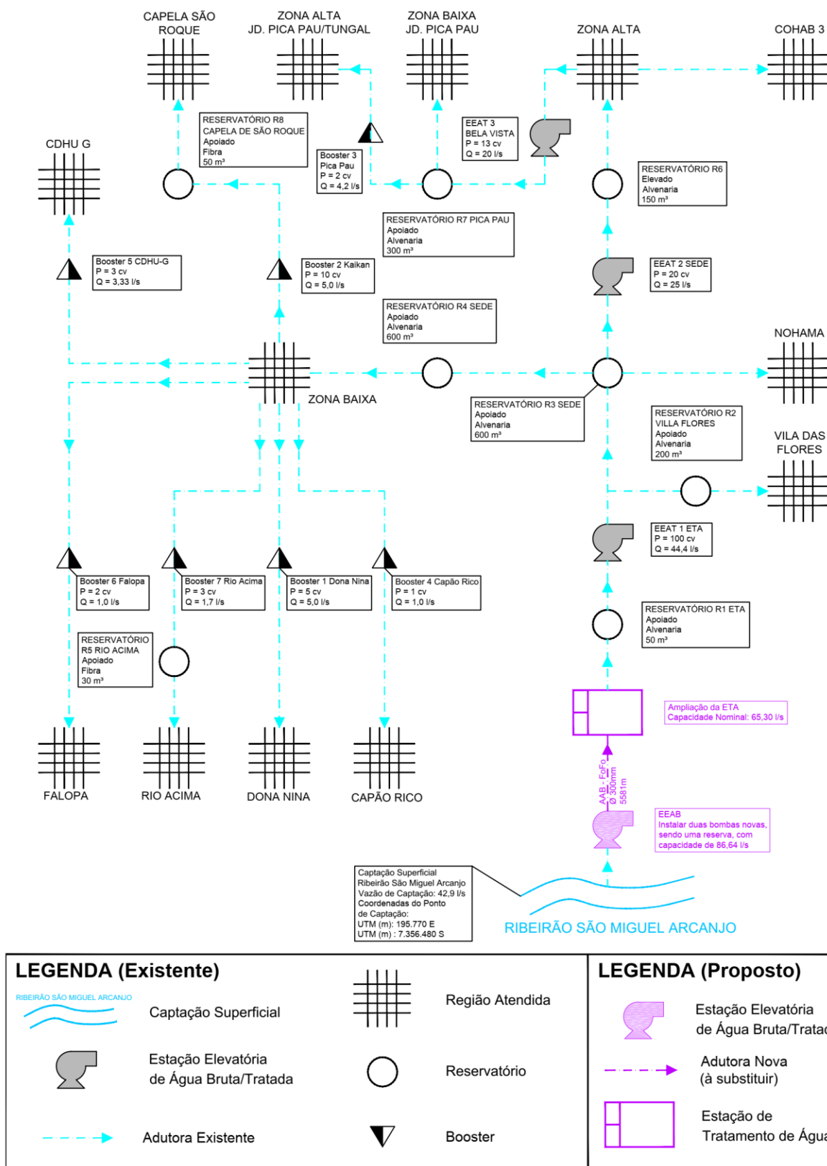
Figura 10.1 – Croqui do Sistema de Abastecimento de Água Proposto para a Sede Urbana
