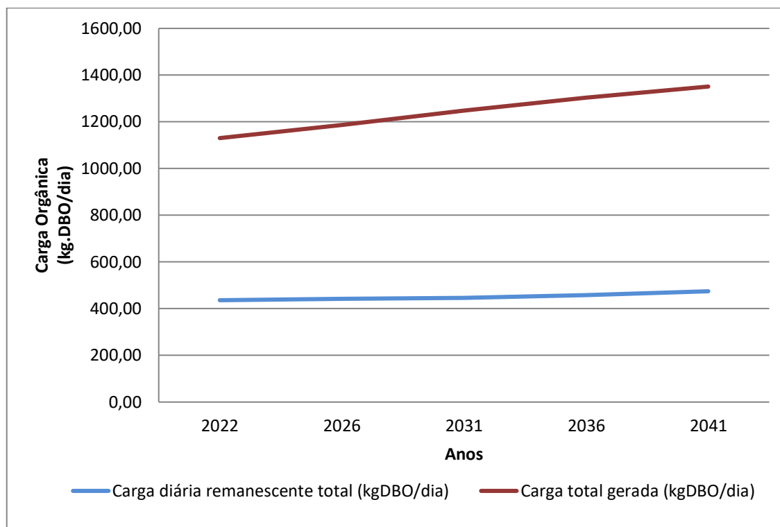
Gráfico 8.12 - Evolução de Cargas Orgânicas (Kg DBO/Dia)
