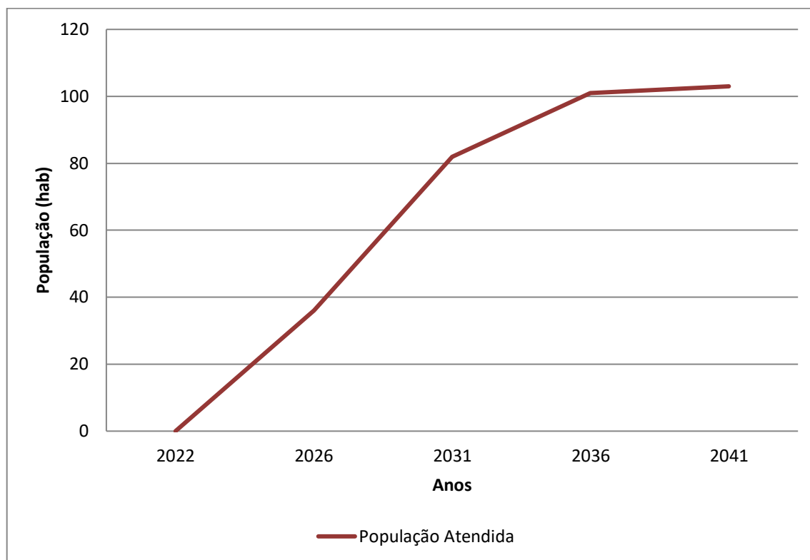
Gráfico 7.12 - População Atendida (hab.) x Anos de Planejamento – Bairro Turvinho
