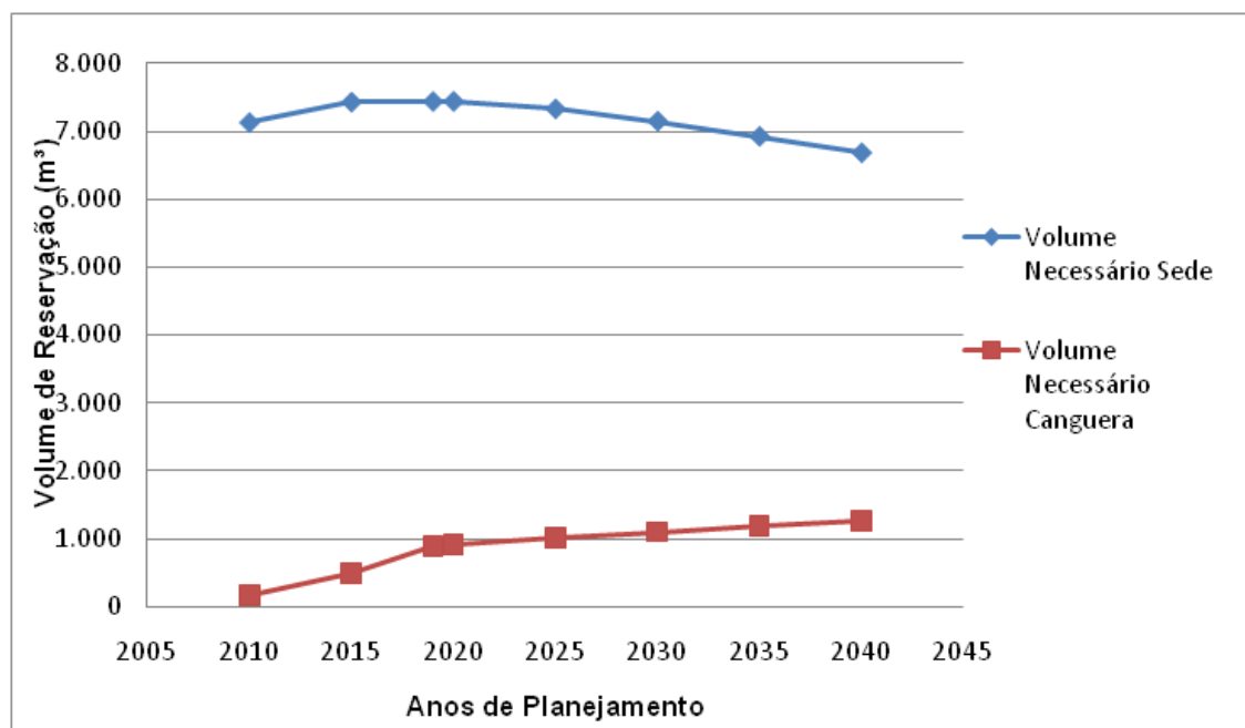
Gráfico 2.4 – Evolução dos Volumes de Reservação Necessários - São Roque
