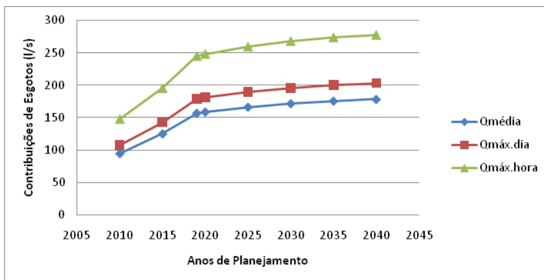
Gráfico 2.6– Evolução das Contribuições de Esgotos – Sede de São Roque
