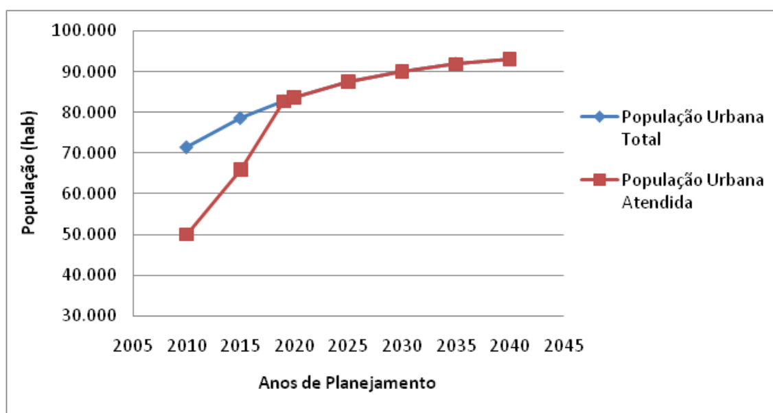
Gráfico 2.5– Populações Urbanas Tratadas (hab) x Anos de Planejamento
