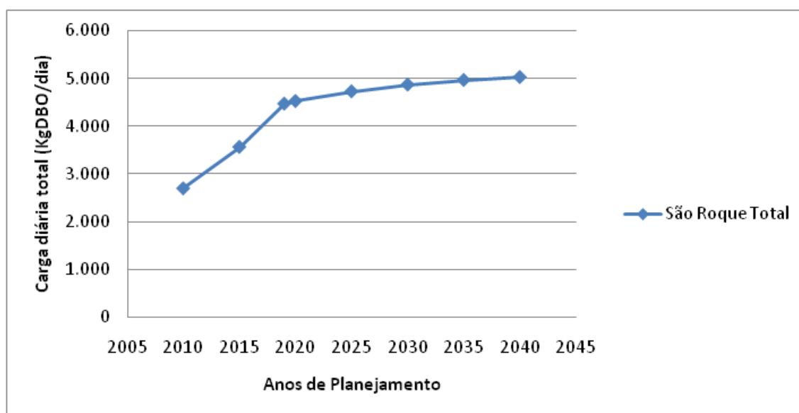
Gráfico 2.7– Evolução das Cargas Orgânicas - Kg DBO/dia
