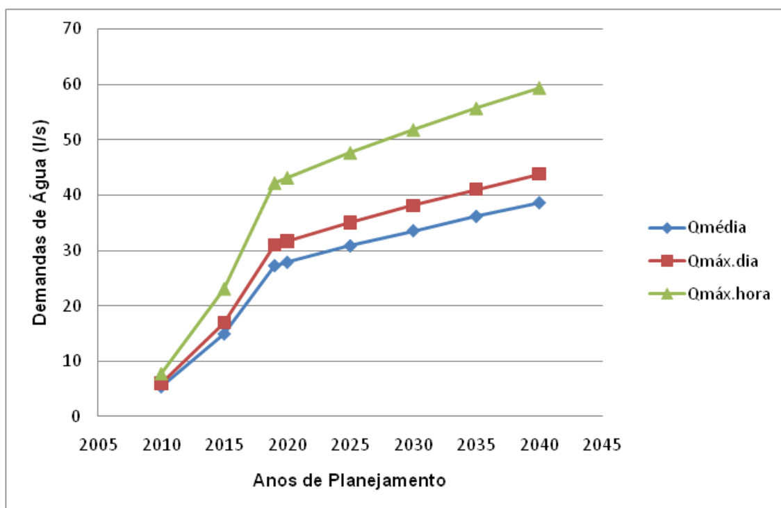
Gráfico 2.3 – Evolução das Demandas – Vazões Disponibilizadas para Distribuição – Canguera
