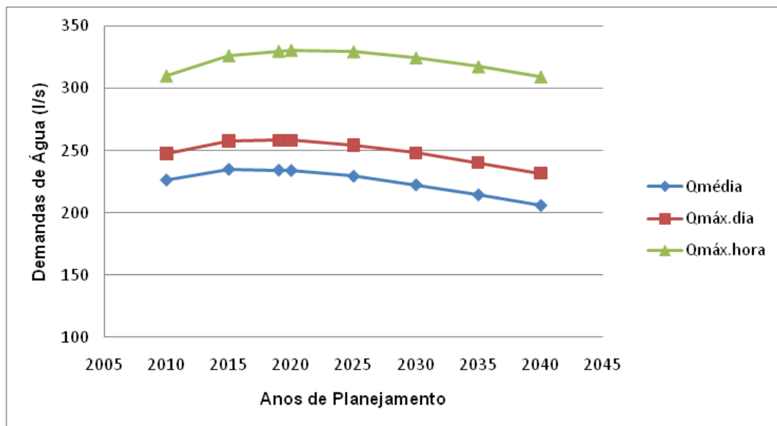
Gráfico 2.2– Evolução das Demandas – Vazões Disponibilizadas para Distribuição – Sede
