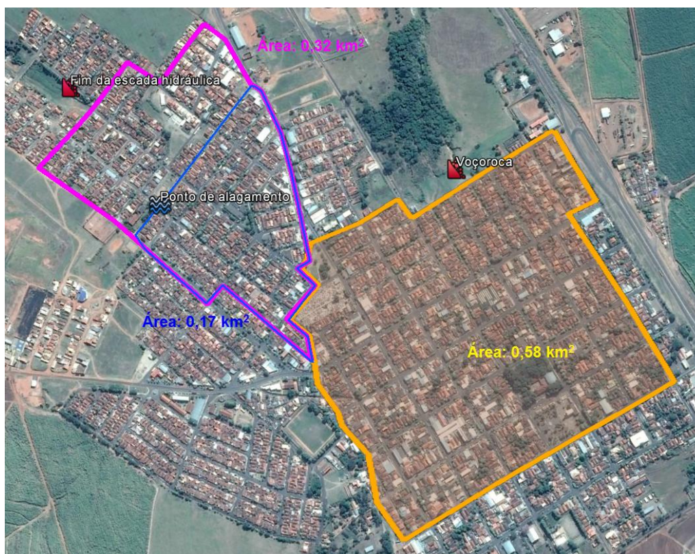
Figura 4.1 - Pontos críticos do sistema de drenagem
