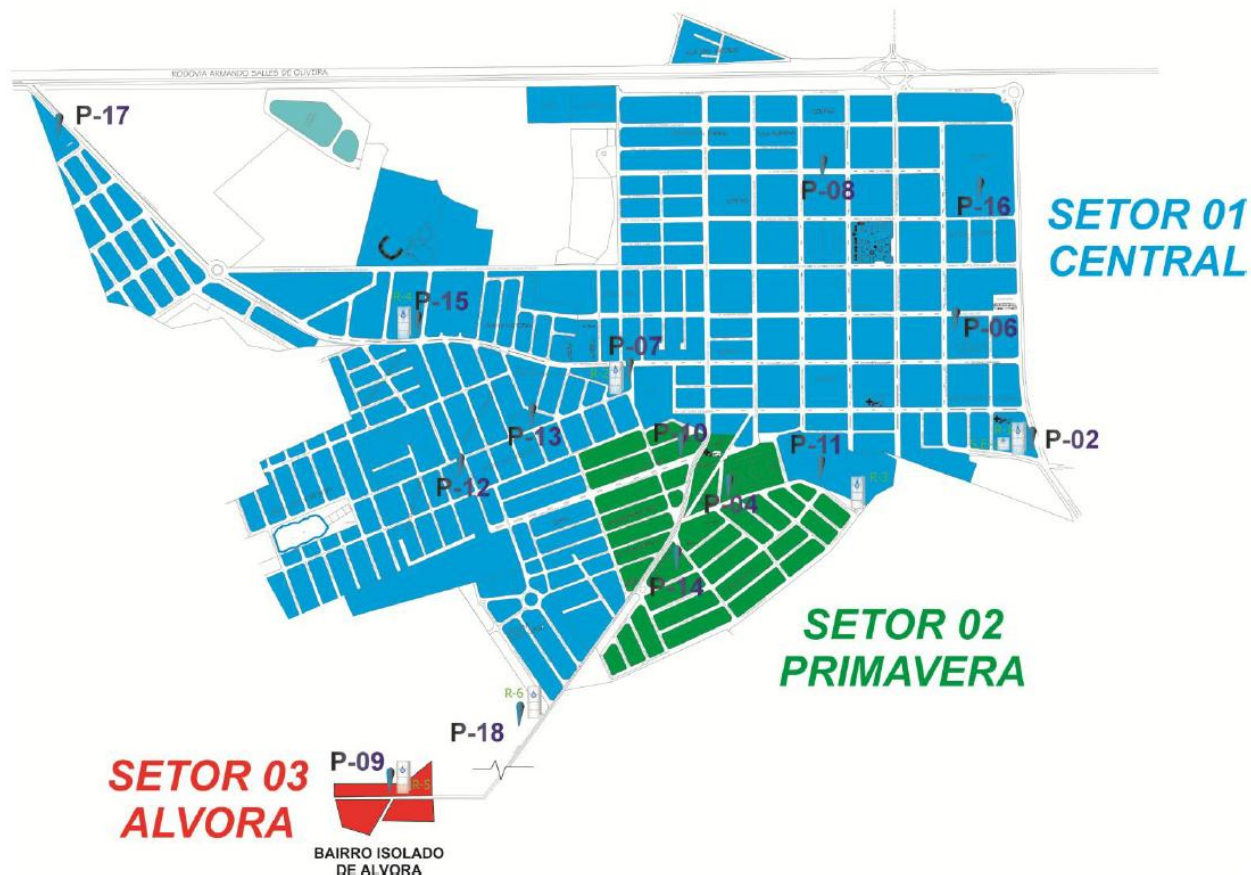
Figura 3.1 – Setores de Distribuição do Sistema de Abastecimento Público de Água
