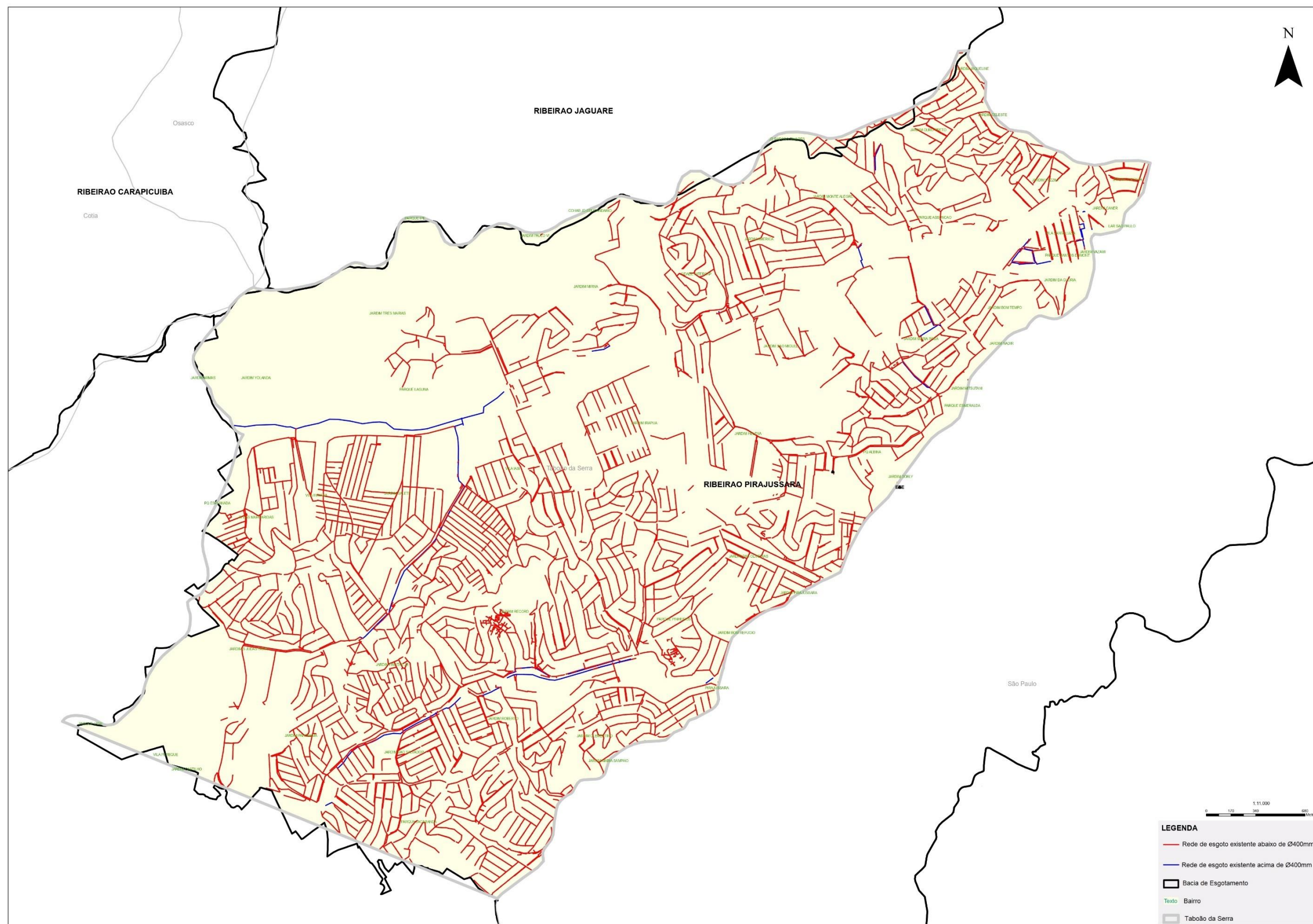
Figura 4.6 – Mapa da Rede Coletora de Esgoto de Taboão da Serra Fonte: SABESP, 2020.
