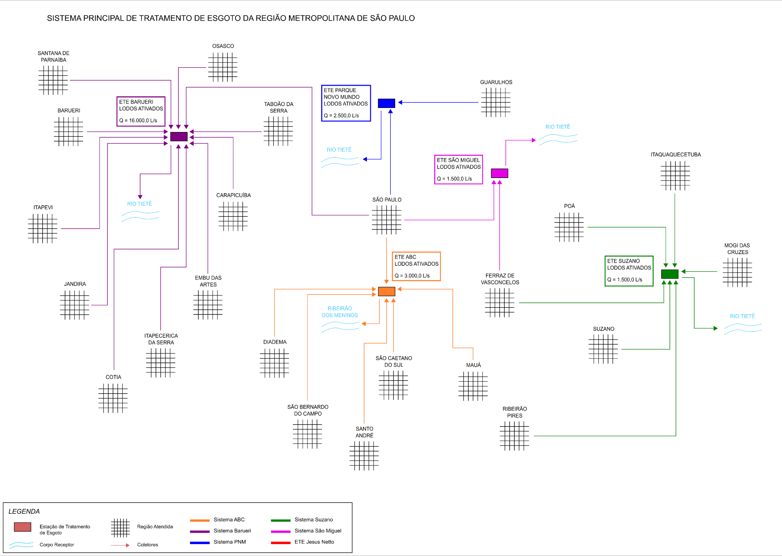
Figura 4.4 – Croqui do Sistema Principal de Tratamento de Esgoto da RMSP Fonte: SABESP, 2020.
