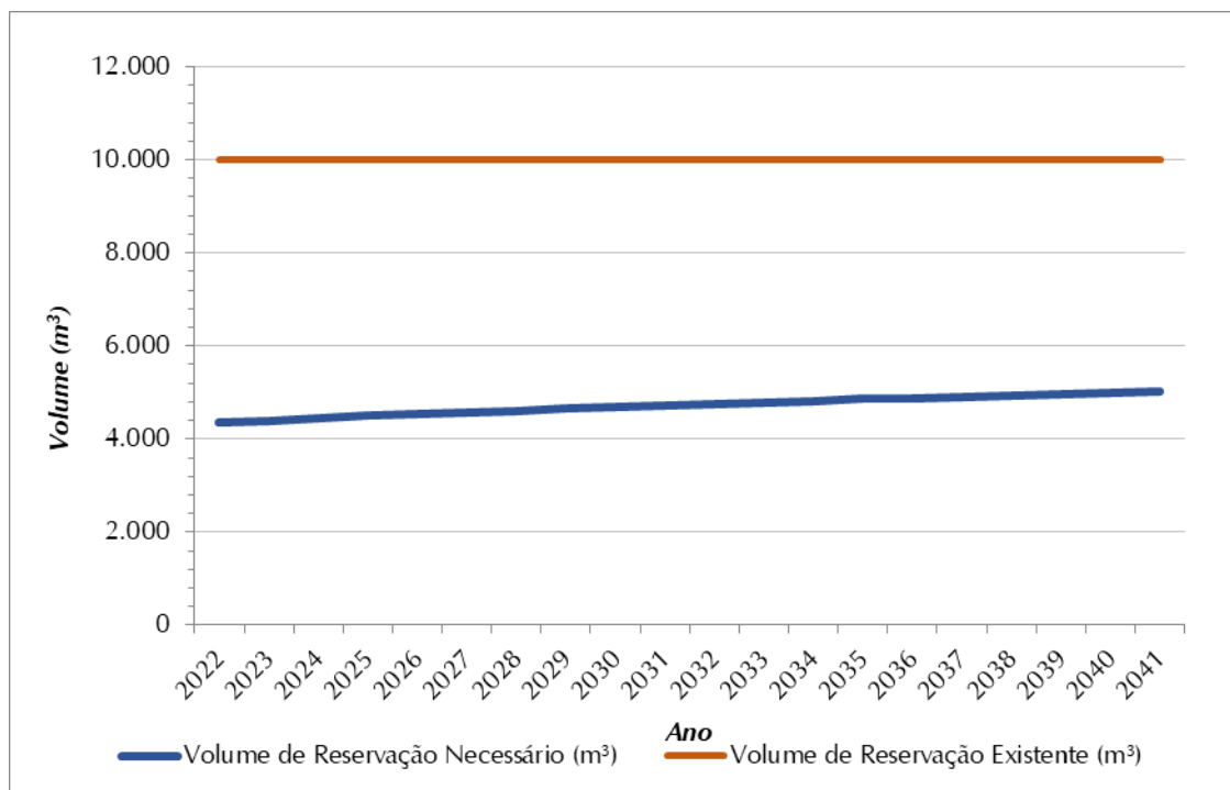
Figura 8.2 - Volume de Reservação Necessário (m³) x Volume de Reservação Atual (m³) - Setor de Abastecimento Centro
