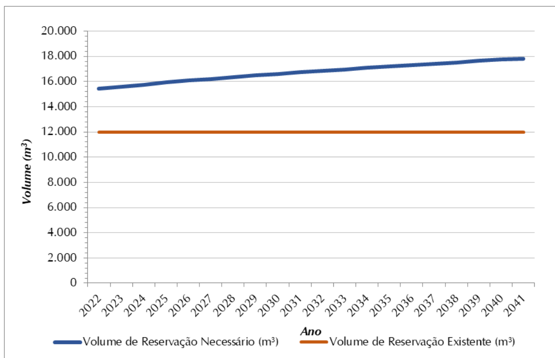
Figura 8.1 - Volume de Reservação Necessário (m³) x Volume de Reservação Atual (m³) - Setor de Abastecimento Jardim Record
