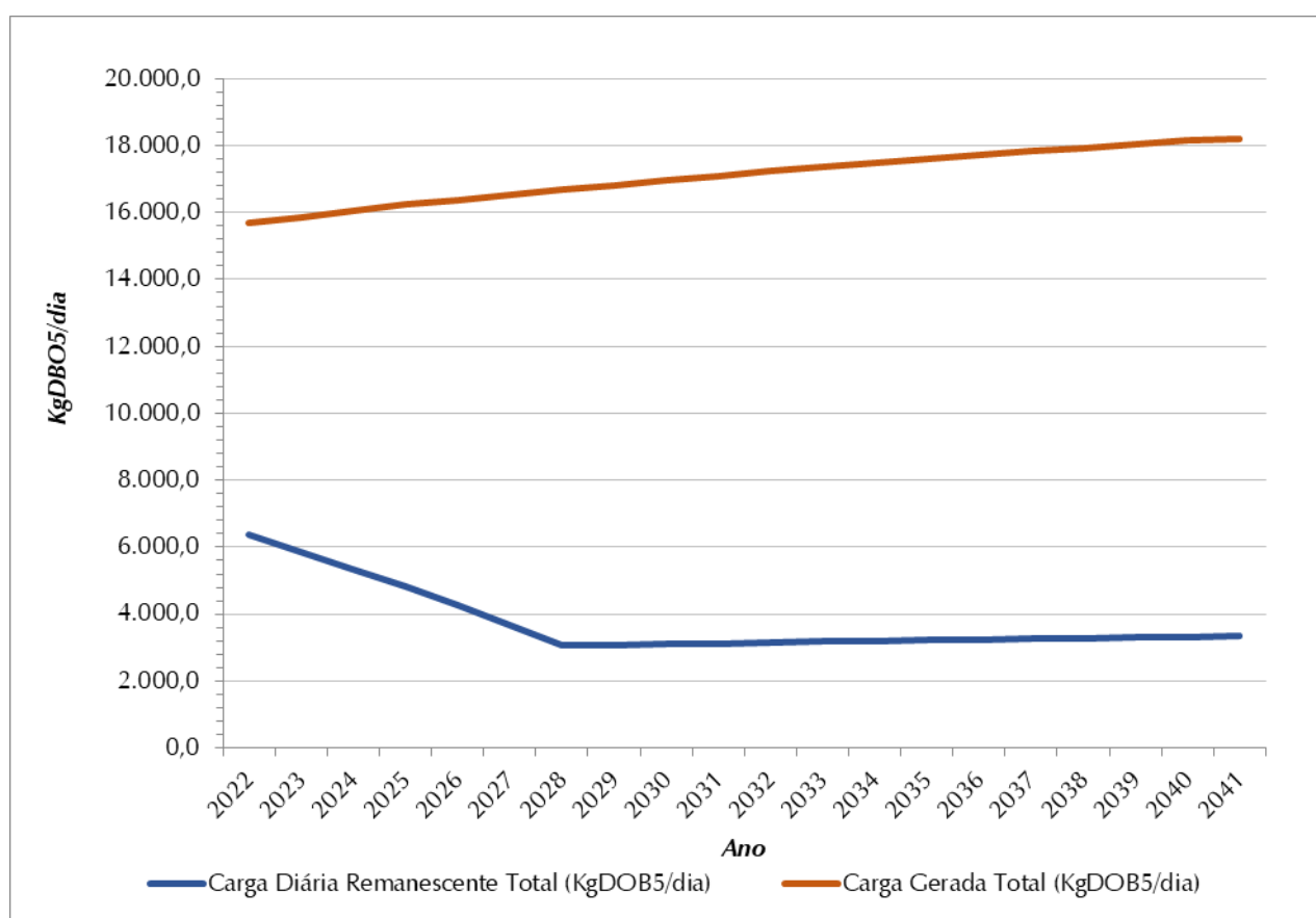
Figura 8.4 - Evolução de Cargas Orgânicas (Kg DBO 5,20 /Dia)
