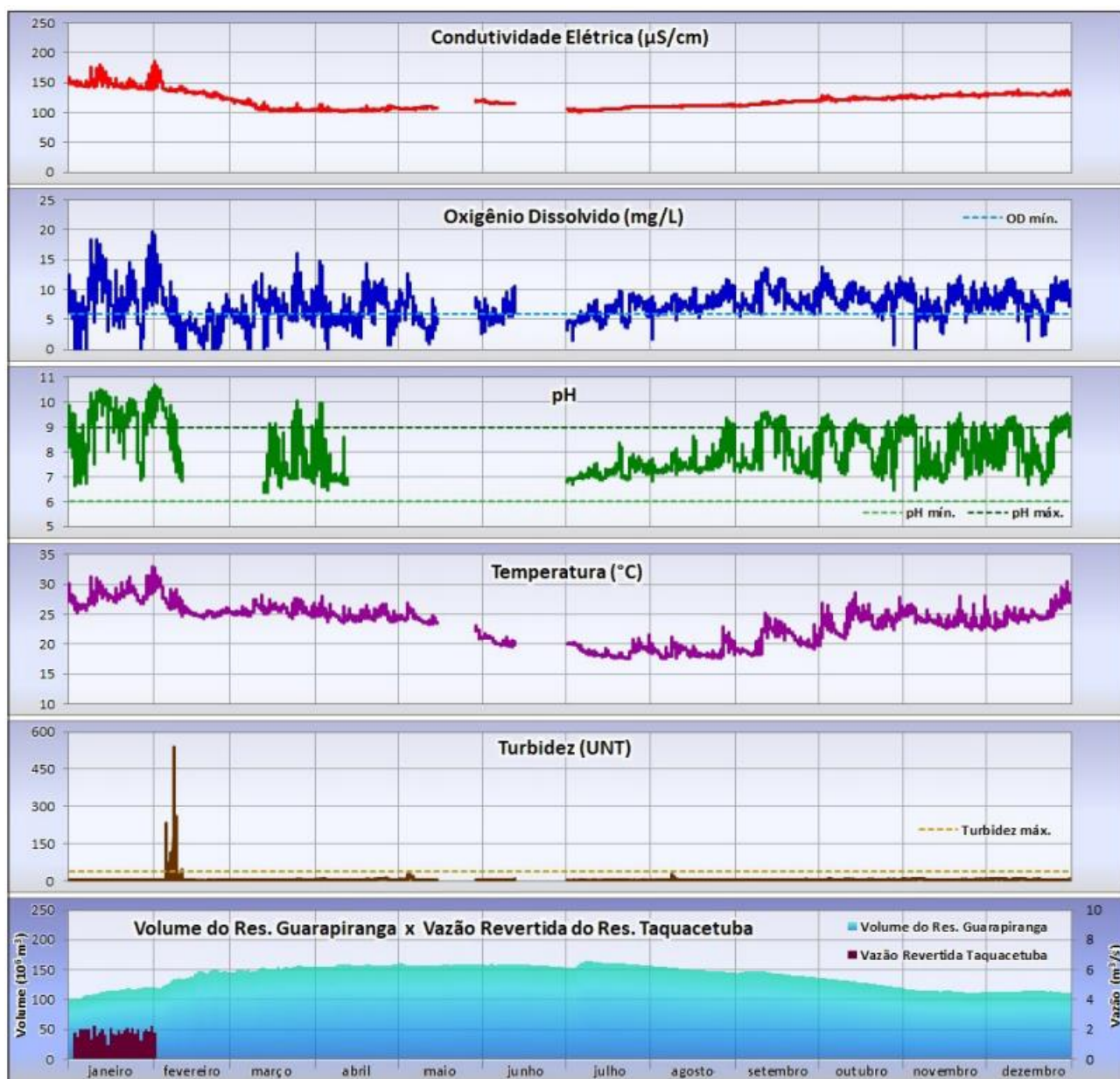
Figura 8.3 - Evolução dos parâmetros medidos pela Estação Automática Guarapiranga de janeiro a dezembro de 2019.
