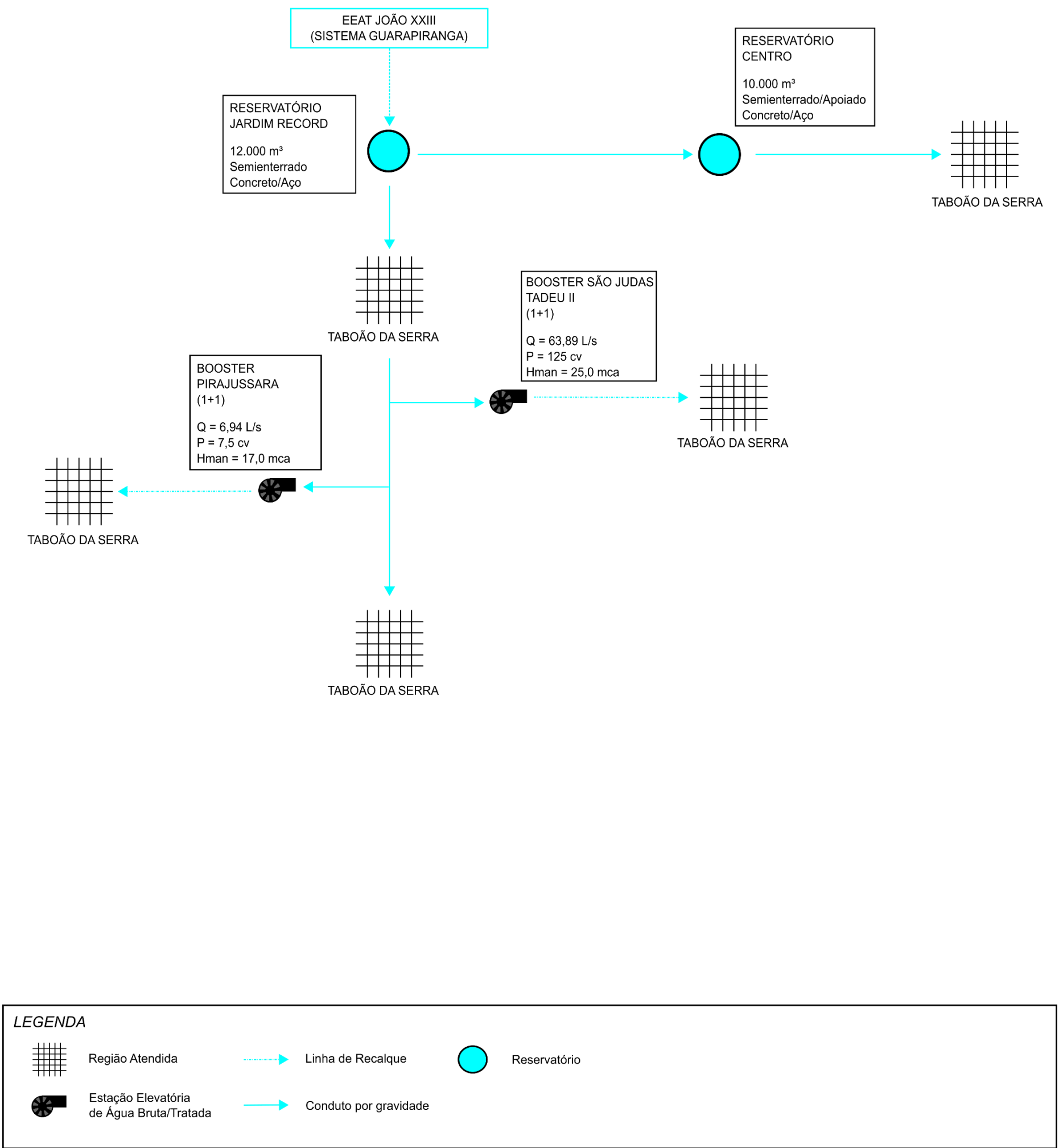
Figura 4.2 – Croqui do Sistema de Abastecimento de Água de Taboão da Serra Fonte: SABESP, 2020.
