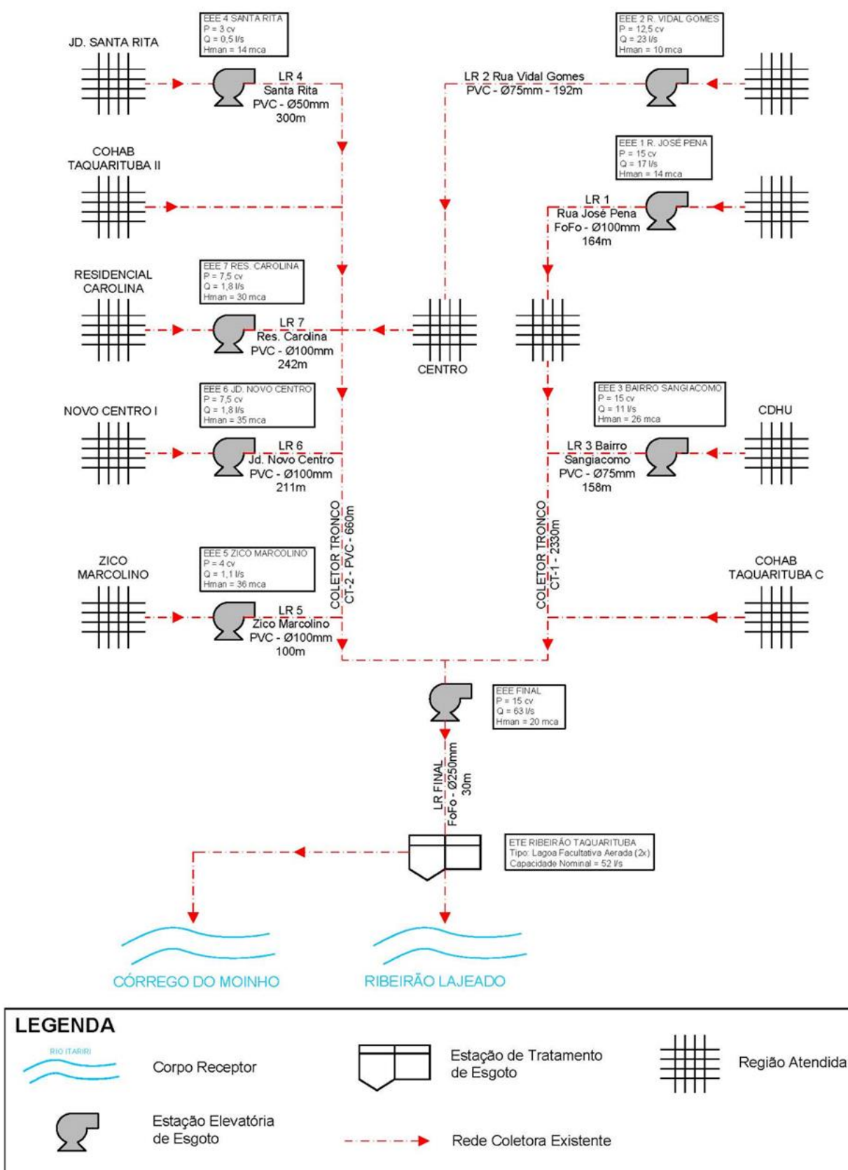
Figura 4.3 – Croqui do Sistema de Esgotamento Sanitário Existente – Sede Urbana
