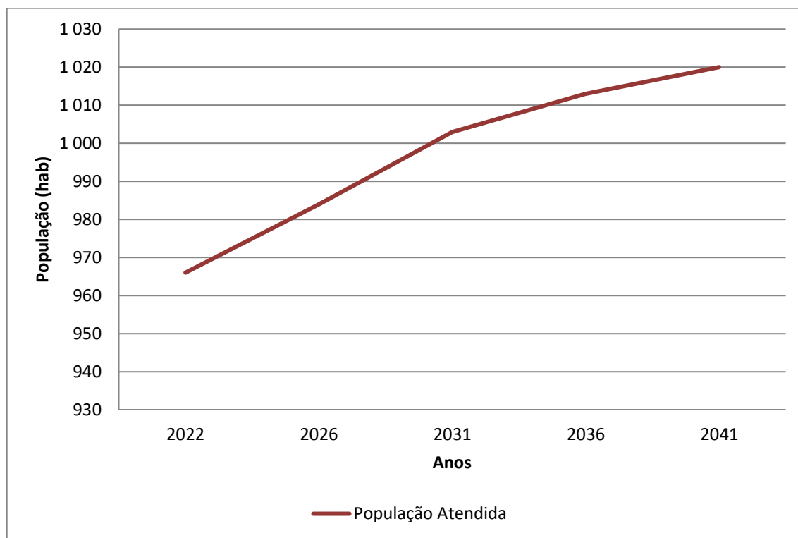
Gráfico 7.5 - População Atendida (hab.) x Anos de Planejamento – Bairro dos Aleixos
