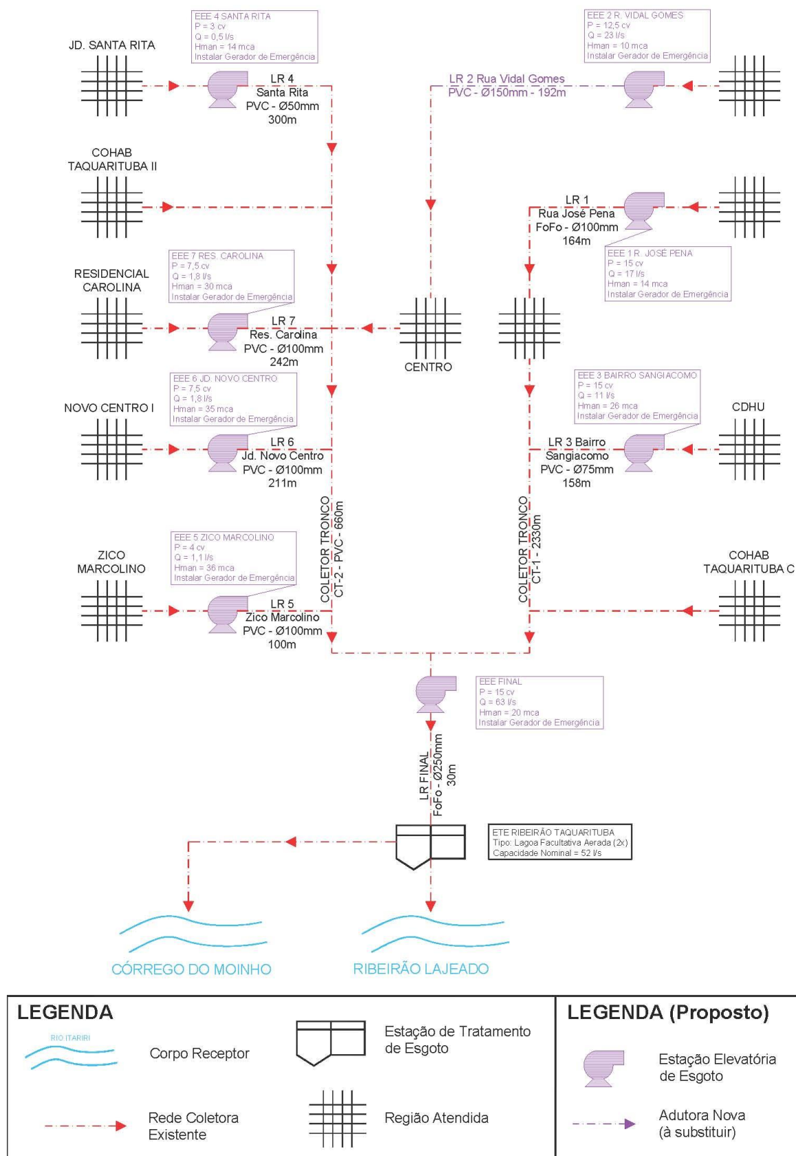
Figura 10.2 – Croqui do Sistema de Esgotamento Sanitário Proposto para o Subsistema da Sede Urbana
