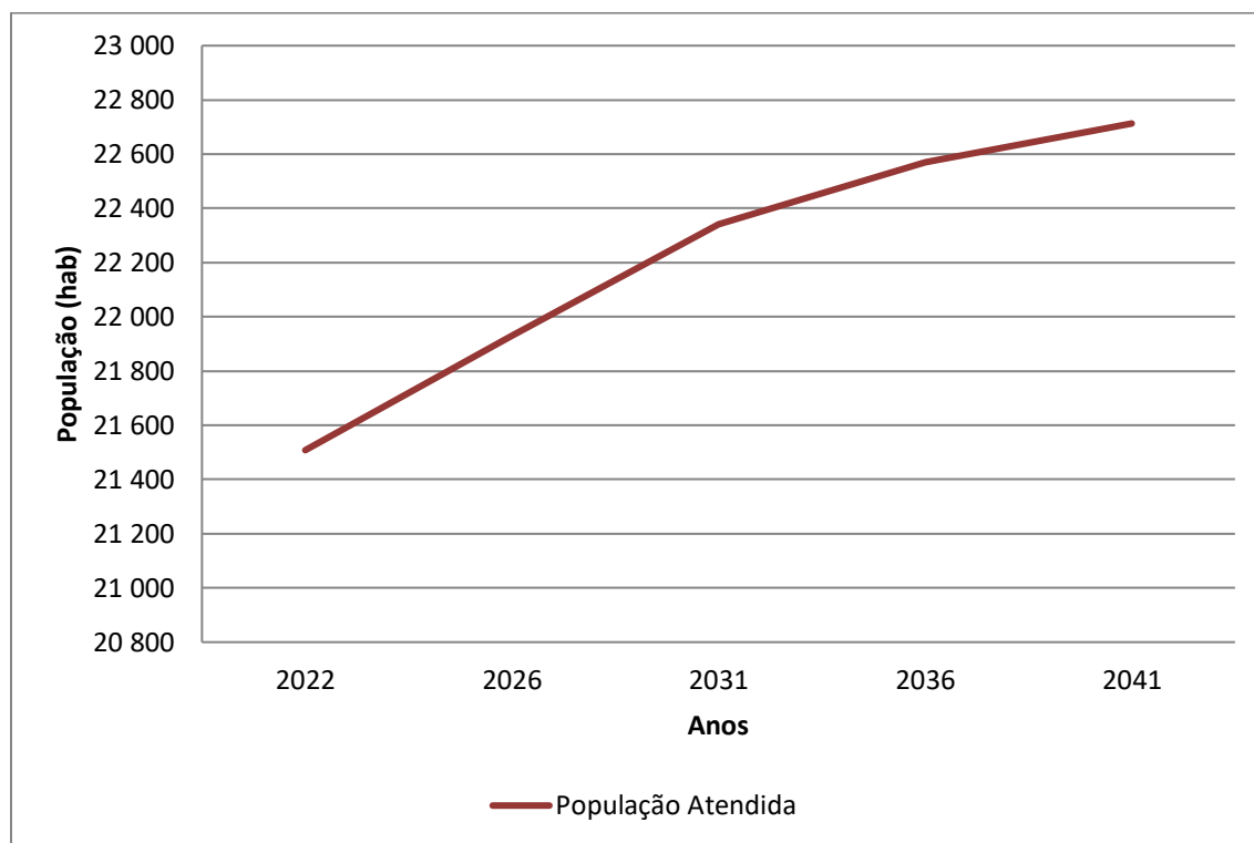
Gráfico 7.2 – População Atendida (hab.) x Anos de Planejamento – Sede Urbana + Bairro dos Aleixos + Bairro Barreiro
