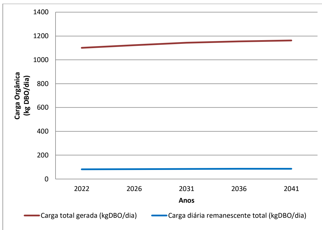
Gráfico 8.6 - Evolução de Cargas Orgânicas (Kg DBO 5 /Dia)
