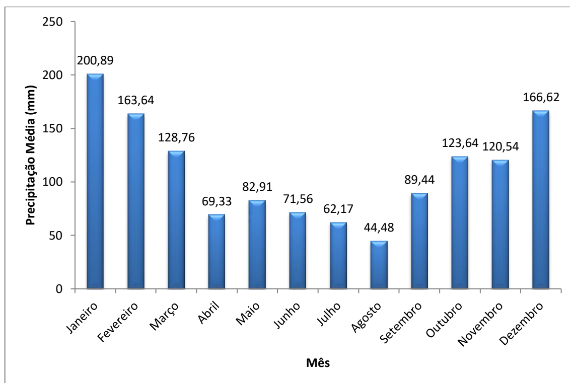
Gráfico 3.1 – Precipitação Média Mensal no Período de 1939 a 2021, Estação E6-013
