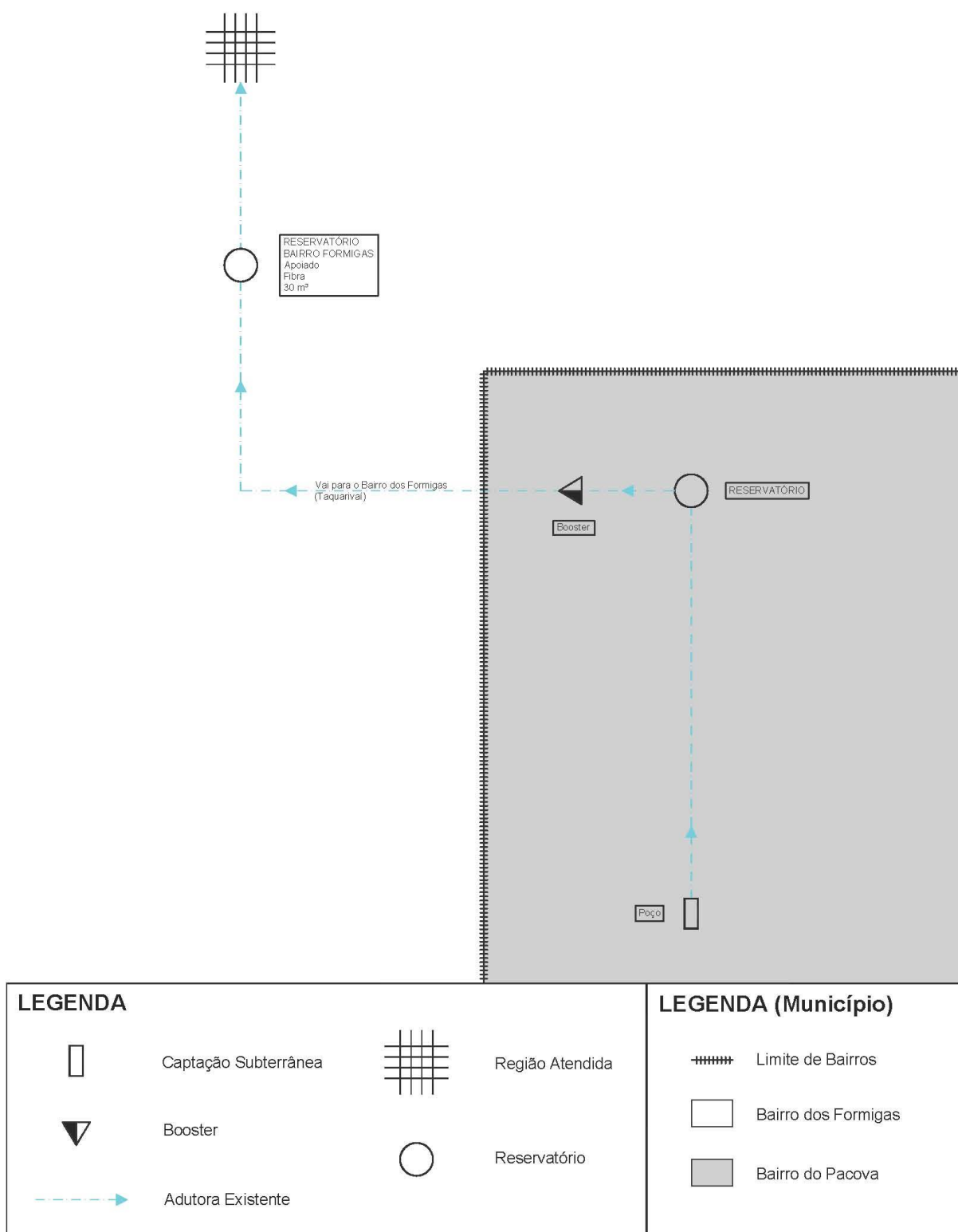
Figura 4.3 – Croqui do Sistema de Abastecimento de Água Existente – Bairro Formigas.
