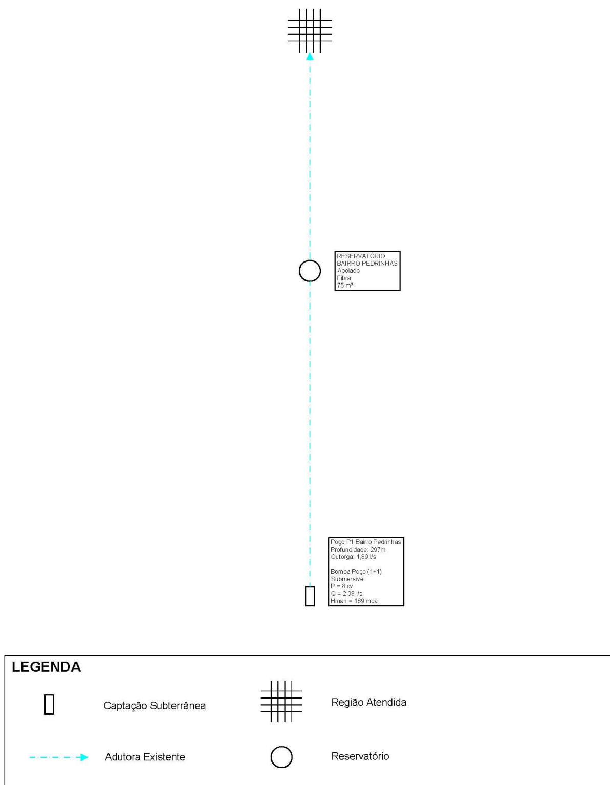
Figura 4.2 – Croqui do Sistema de Abastecimento de Água Existente – Bairro Pedrinhas.
