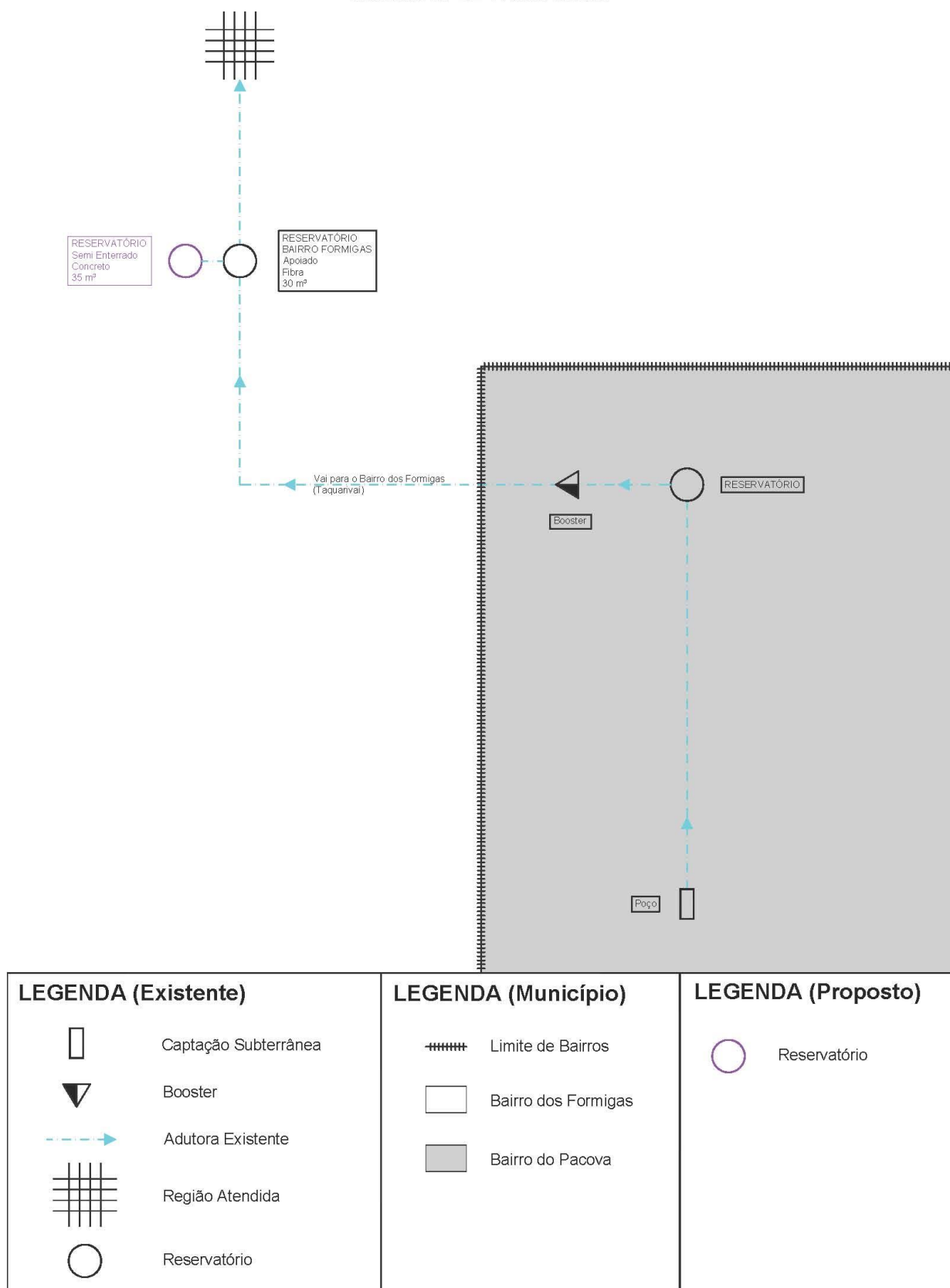
Figura 10.2 – Croqui do Sistema de Abastecimento de Água Proposto para o Bairro Formigas
