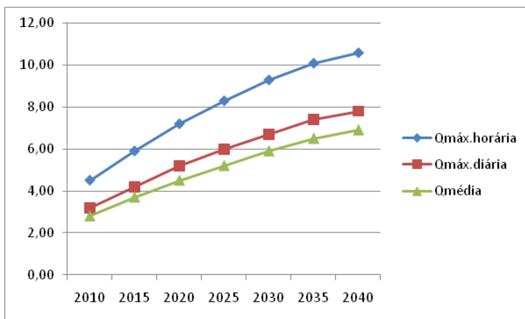
Gráfico 2.5 – Contribuições de Esgotos (l/s)x Anos de Planejamento
