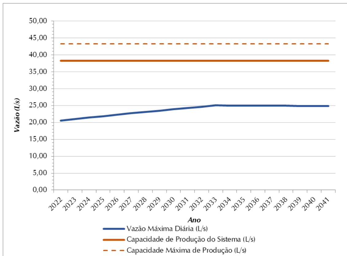
Figura 8.1 – Demandas Máximas Diárias (L/s) X Vazão Captada (L/s) – SAA Sede
