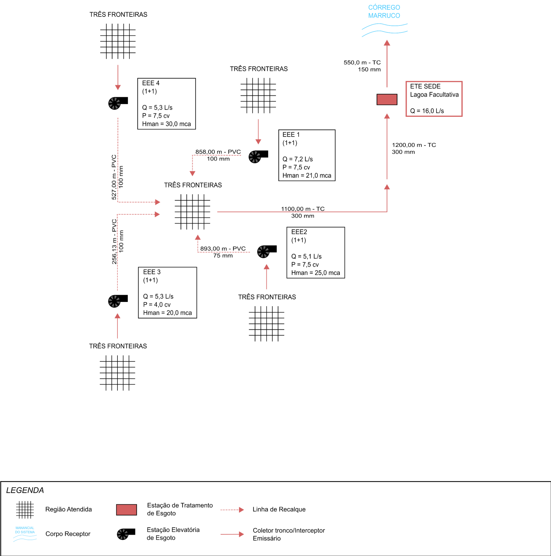
Figura 4.2 – Croqui do Sistema de Esgotamento Sanitário da Sede de Três Fronteiras
