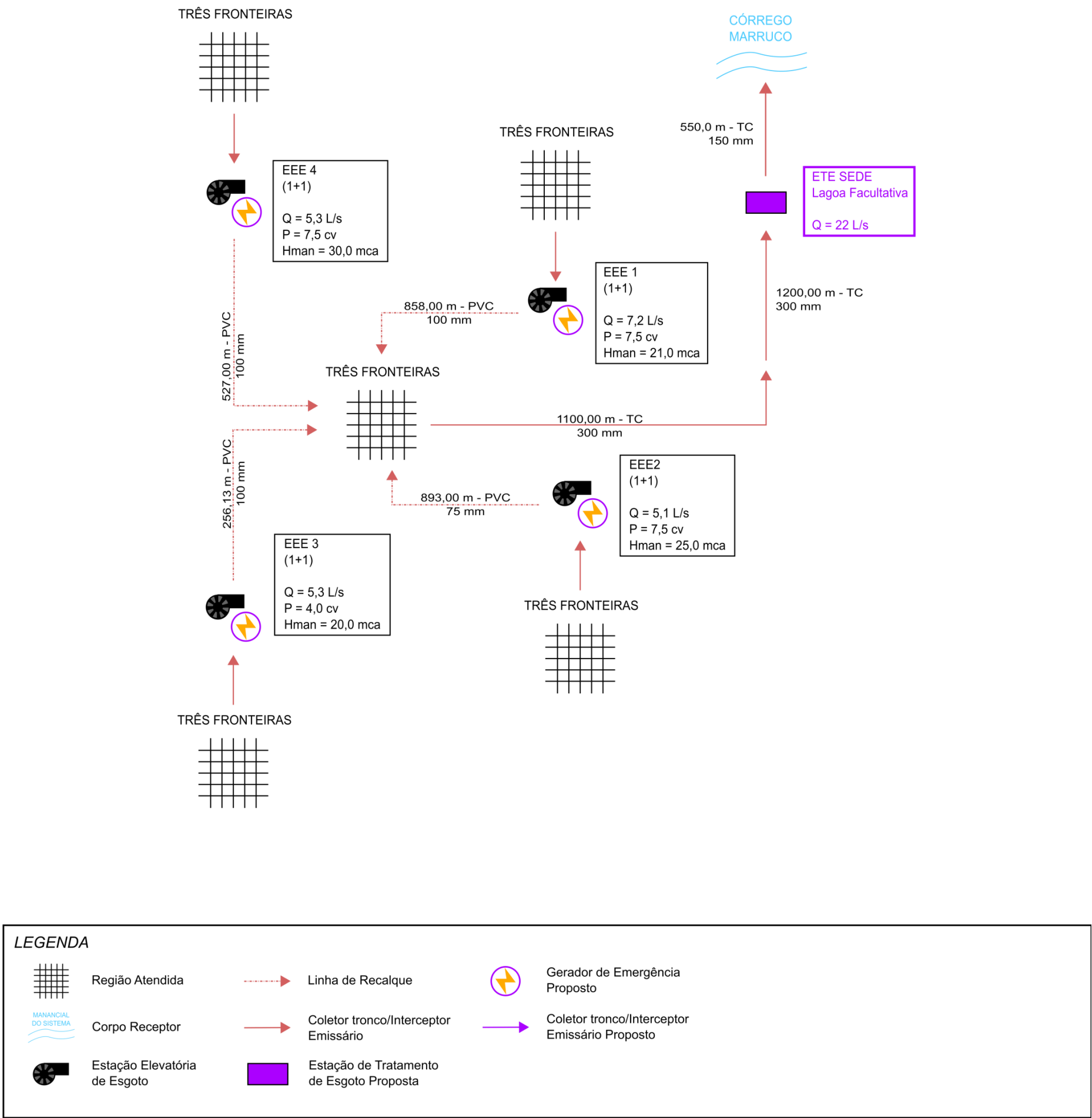
Figura 10.2 – Croqui das intervenções propostas para o sistema de esgotamento sanitário Sede
