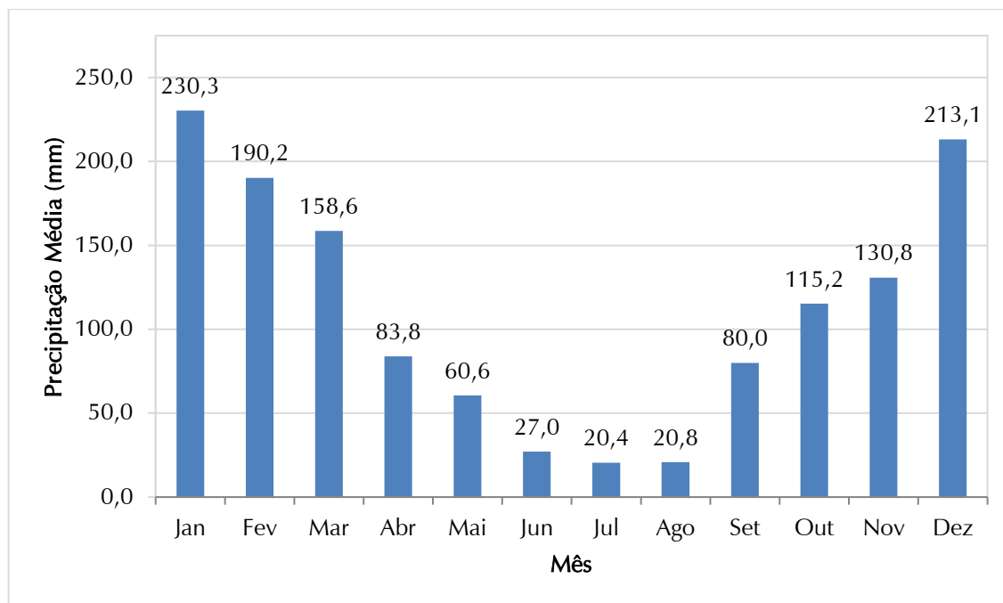
Figura 3.2 - Precipitação Média Mensal no Período de 1968 a 2001, Estação B7-016
