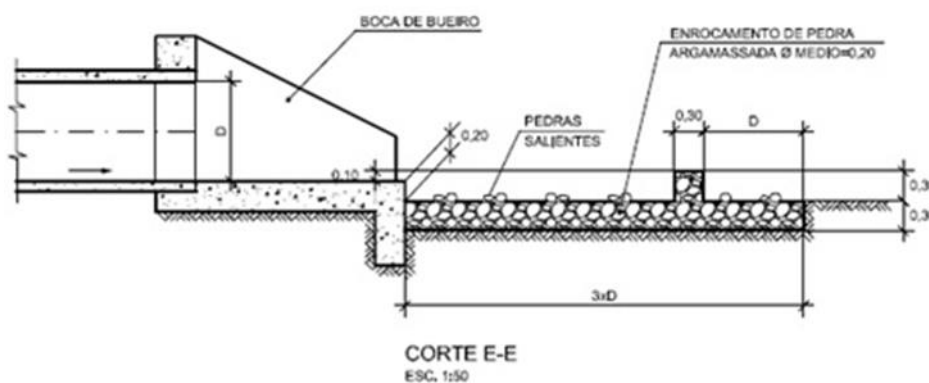
Ilustração 8.7 –Dissipador
