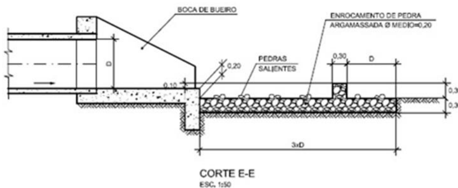
Ilustração 8.3 – Dissipador
