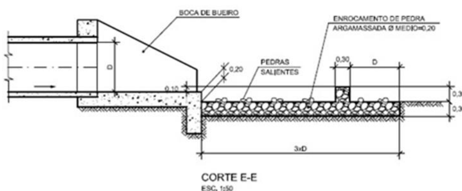
Ilustração 8.5 – Dissipador
