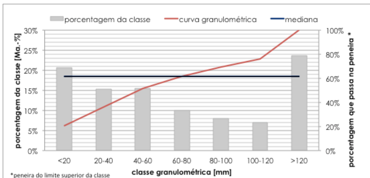
Figura 32 – Curva do peneiramento por classes granulométricas
