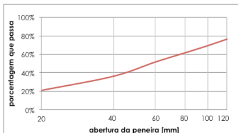
Figura 33 – Curva granulométrica
