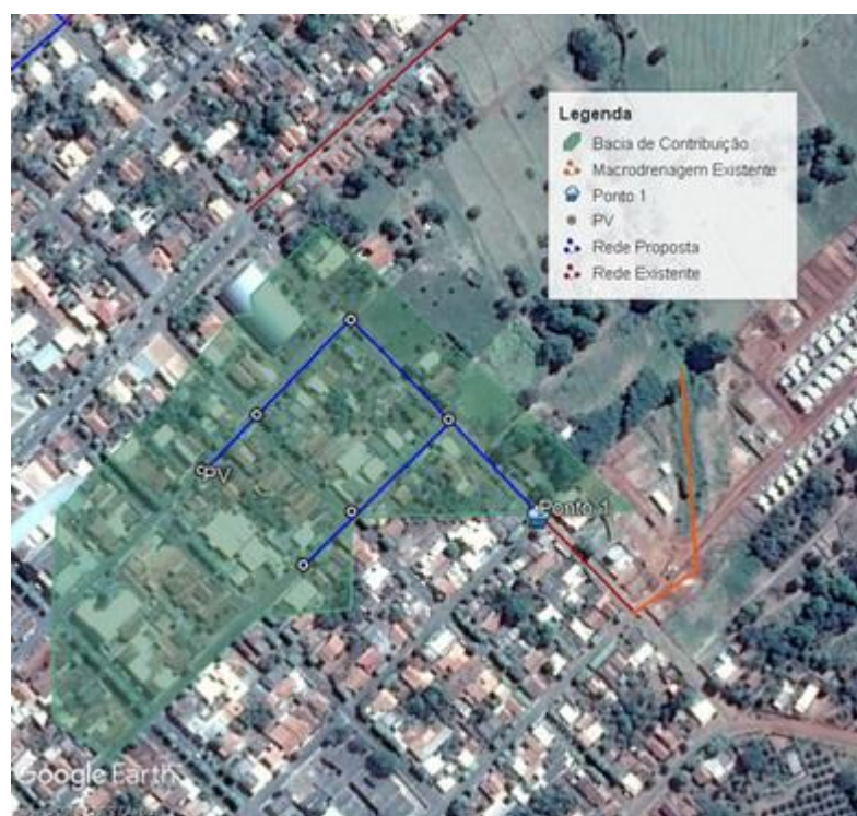
Ilustração 8.1- Intervenções propostas para o ponto de alagamento 1.
