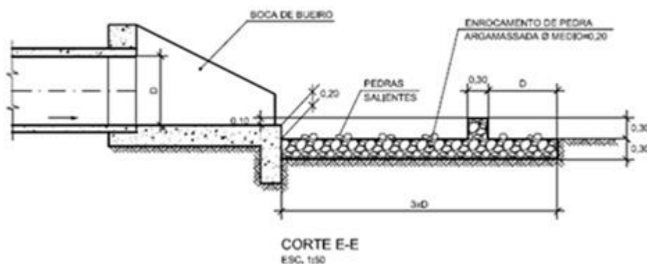
Ilustração 8.4- Dissipador.
