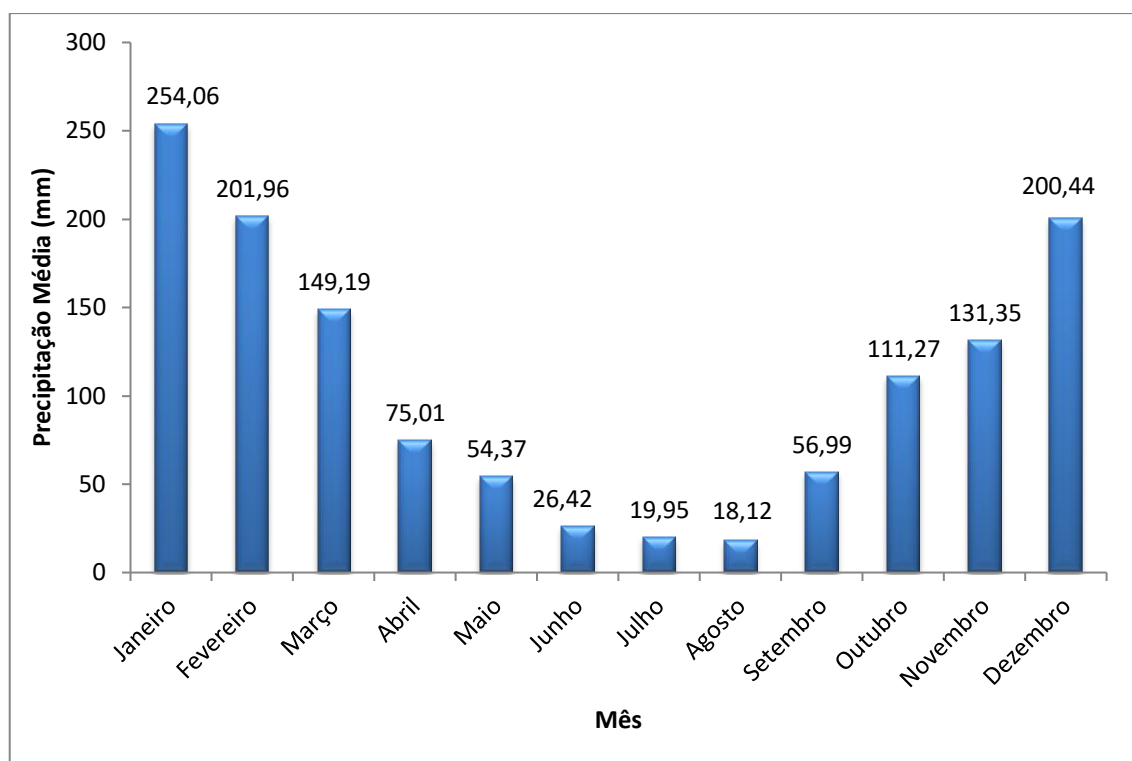
Gráfico 3.1 – Precipitação Média Mensal no Período de 1970 a 2021, Estação B7-011
