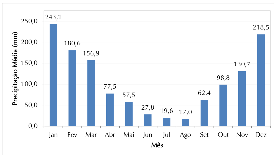
Figura 3.2 – Precipitação Média Mensal no Período de 1970 a 2021, Estação B7-041
