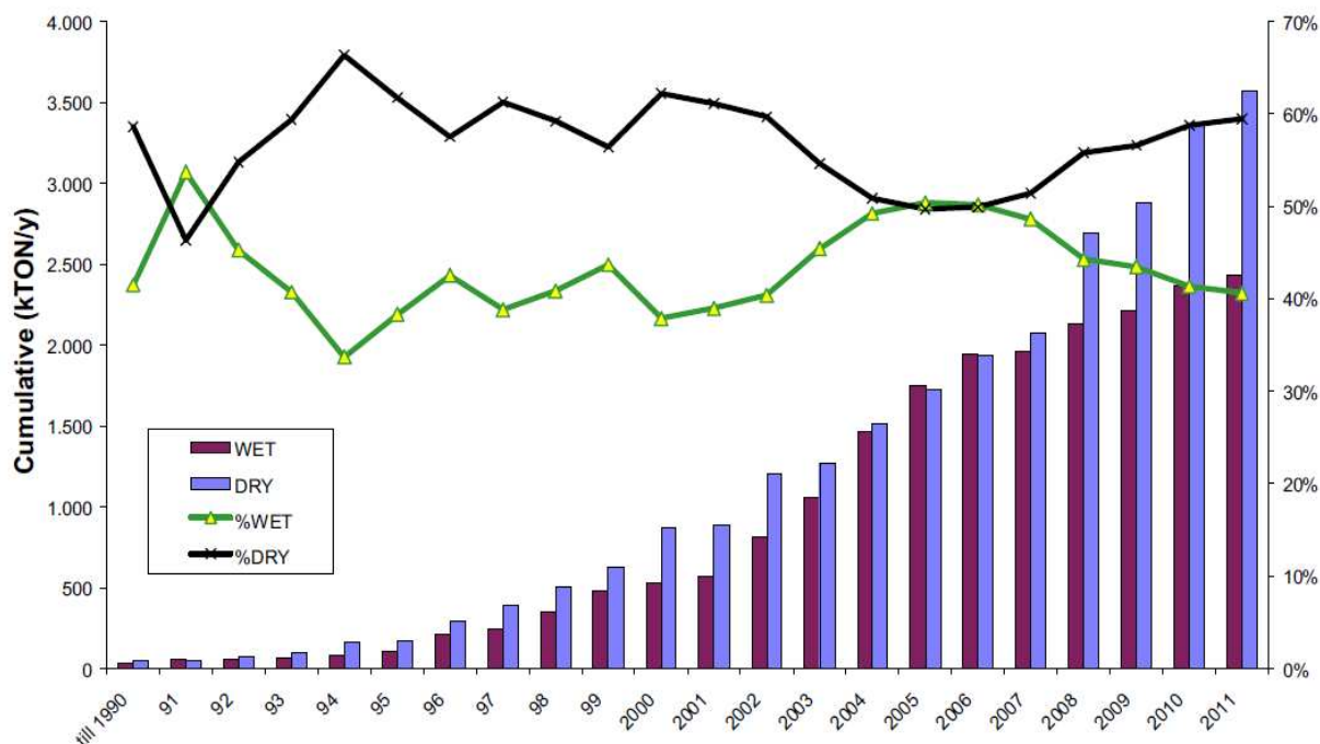
Figura 155: Desenvolvimento de tecnologias de fermentação secas e úmidas na Europa.
