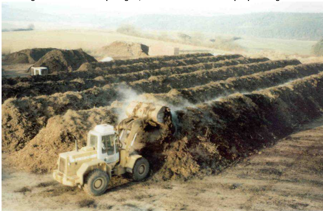
Figura 162: Leira de compostagem, sendo montada e revirada por pá-carregadeira.
