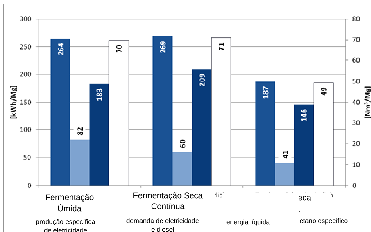
Figura 159: Balanço energético no processo termofílico para fermentação úmida, seca contínua e fermentação seca descontínua.
