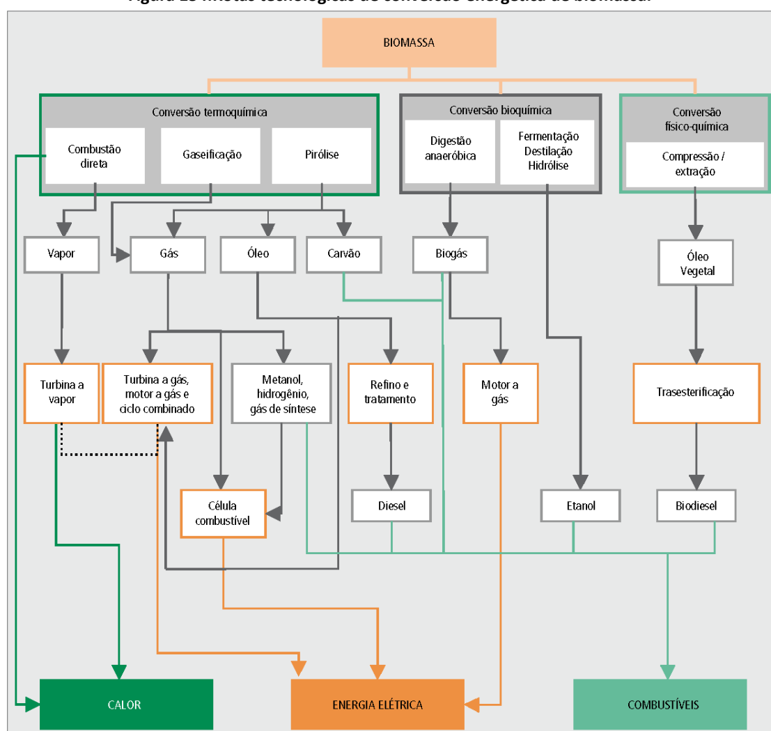
Figura 154: Rotas tecnológicas de conversão energética de biomassa.
