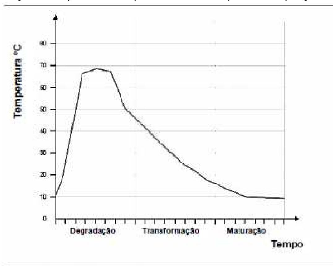
Figura 161:Variação do nível de temperatura na leira durante o processo de compostagem.
