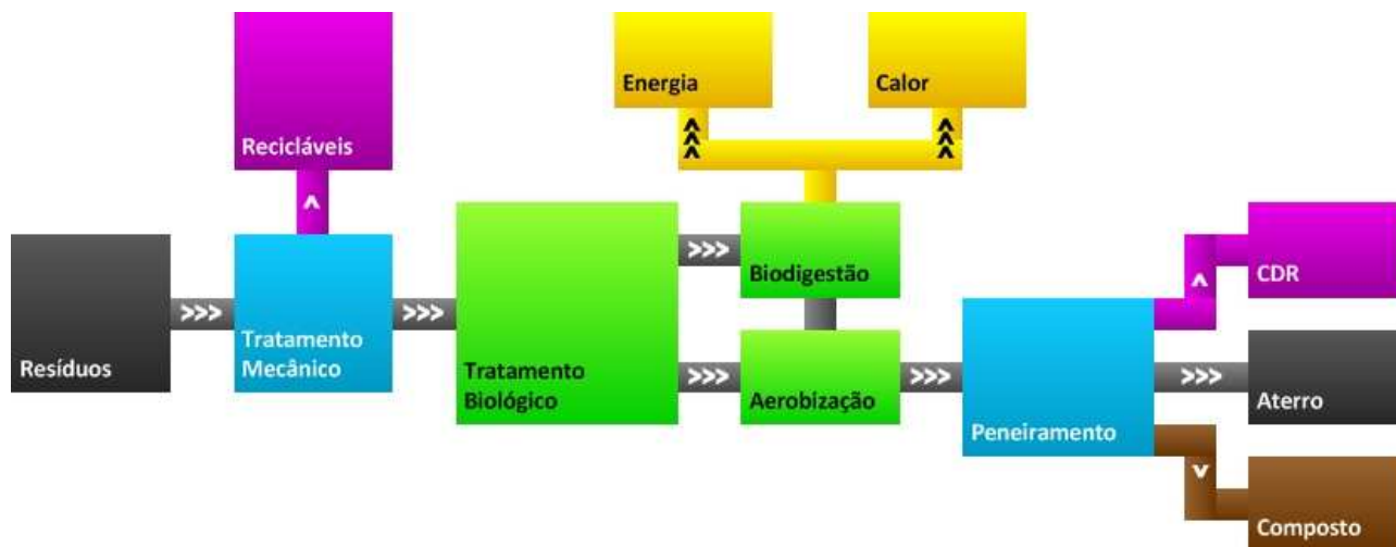
Figura 176: Fases do processo.
