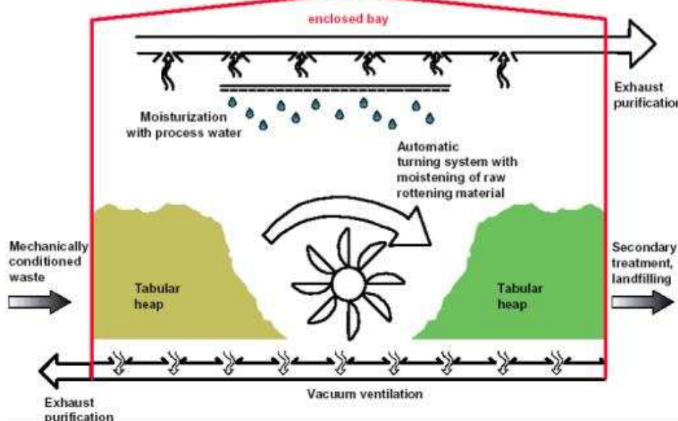
Figura 170: Perfil da leira de compostagem tabular.
