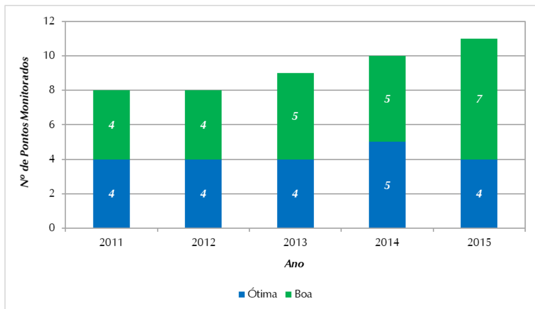
Figura 2.1 – Resultados IQA na UGRHI 19 entre 2011 e 2015
